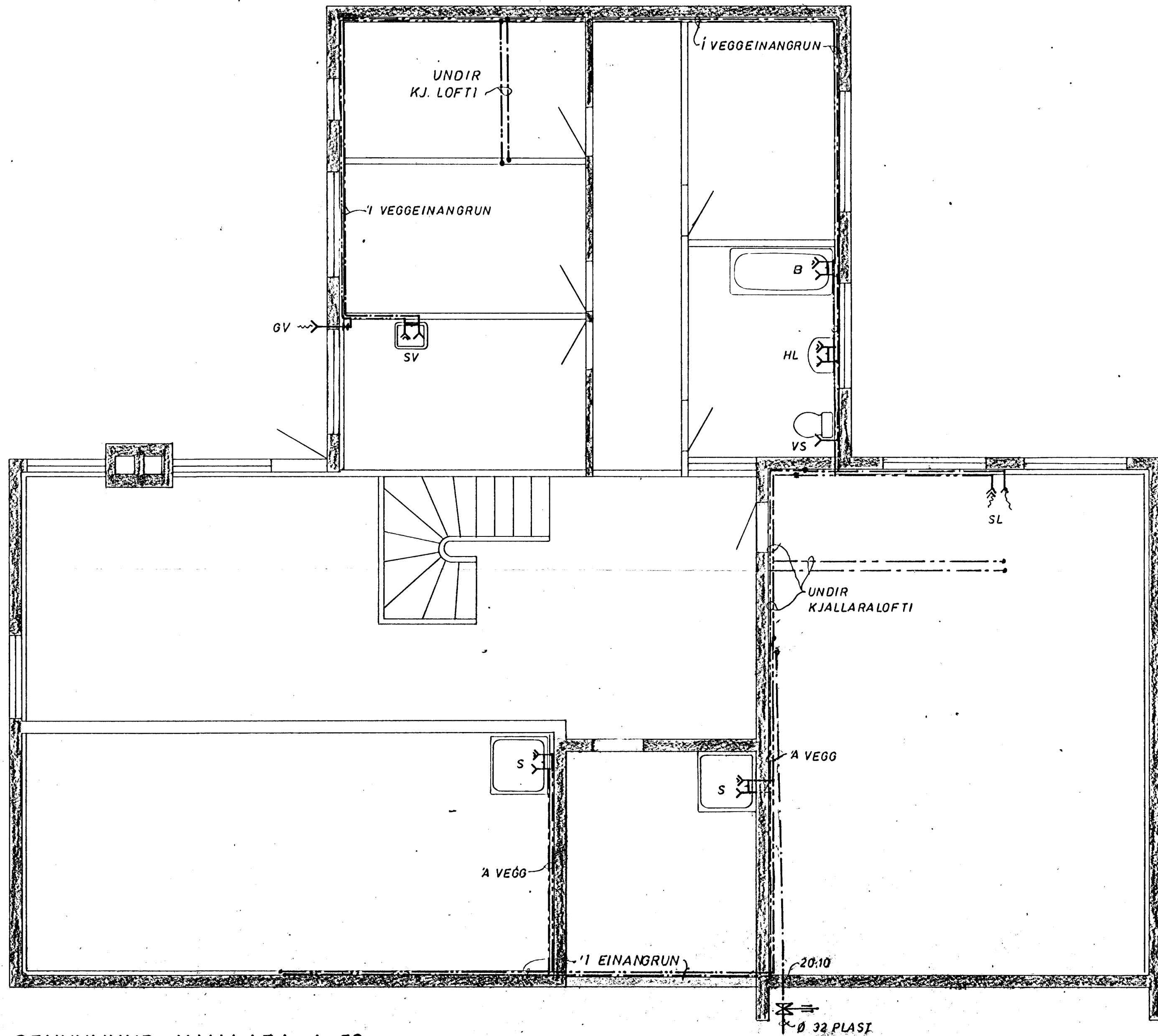
GRUNNMYND KJALLARA 1: 50
