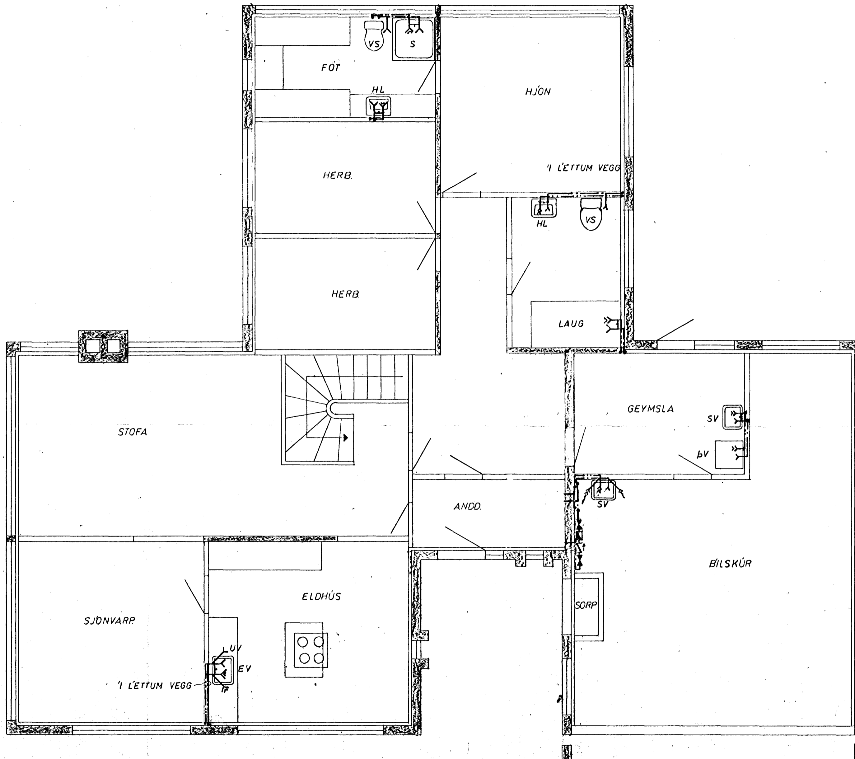
GRUNNMYND HÆÐAR 1:50
