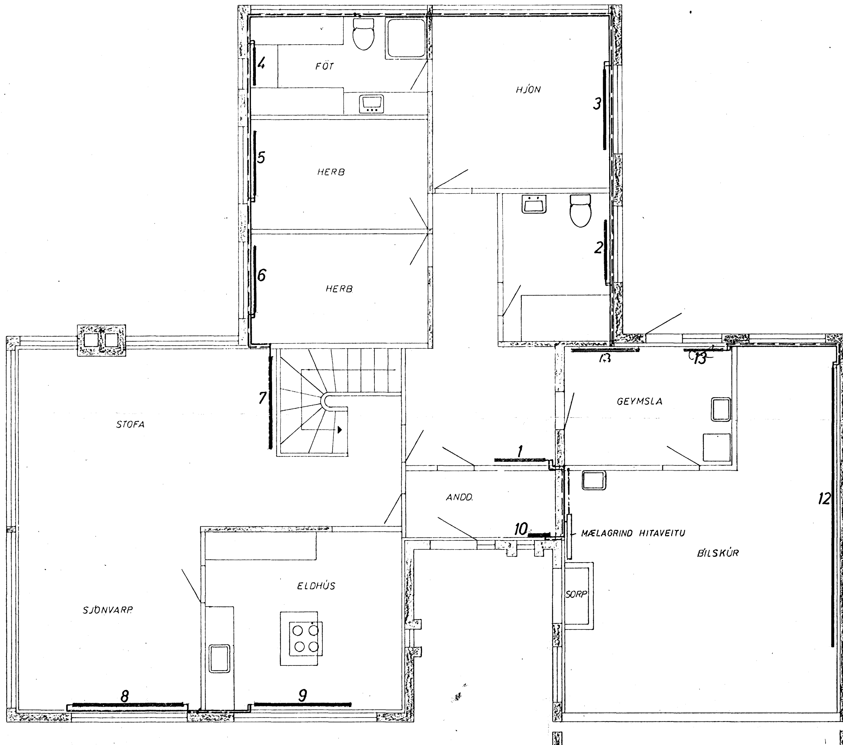
GRUNNMYND HÆÐAR 1: 50
