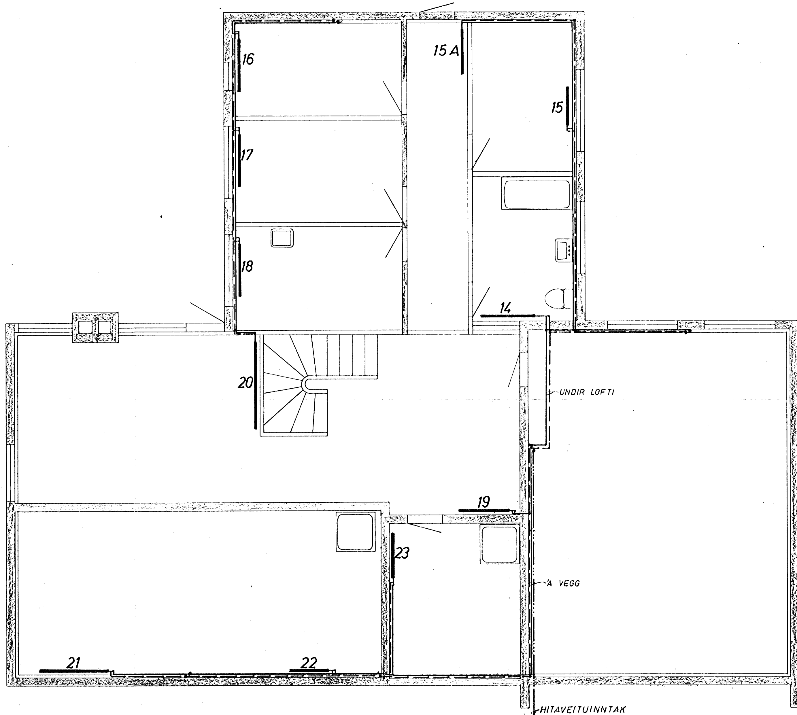
GRUNNMYND KJALLARA 1: 50
