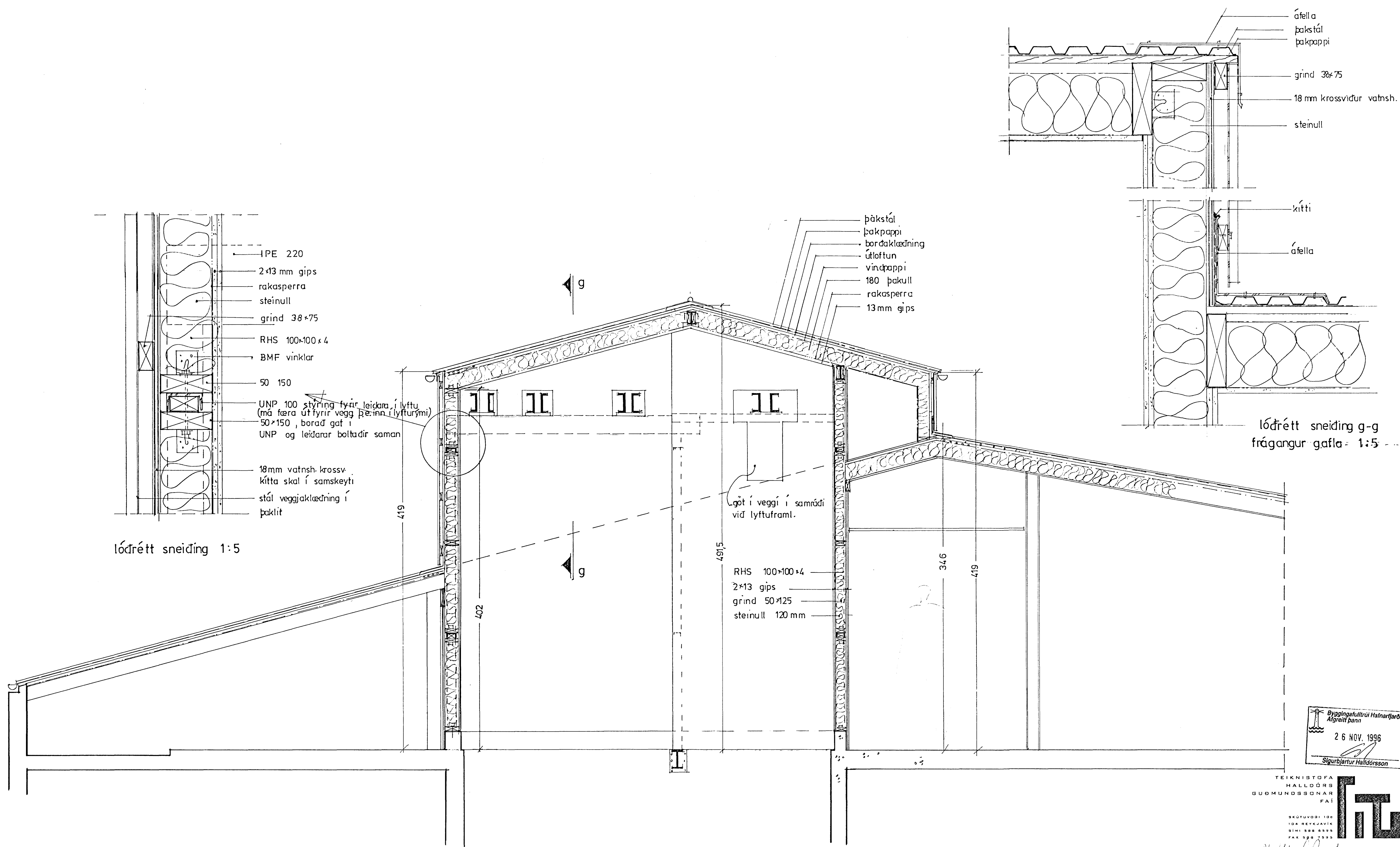
sneiðing b-b 1:20
