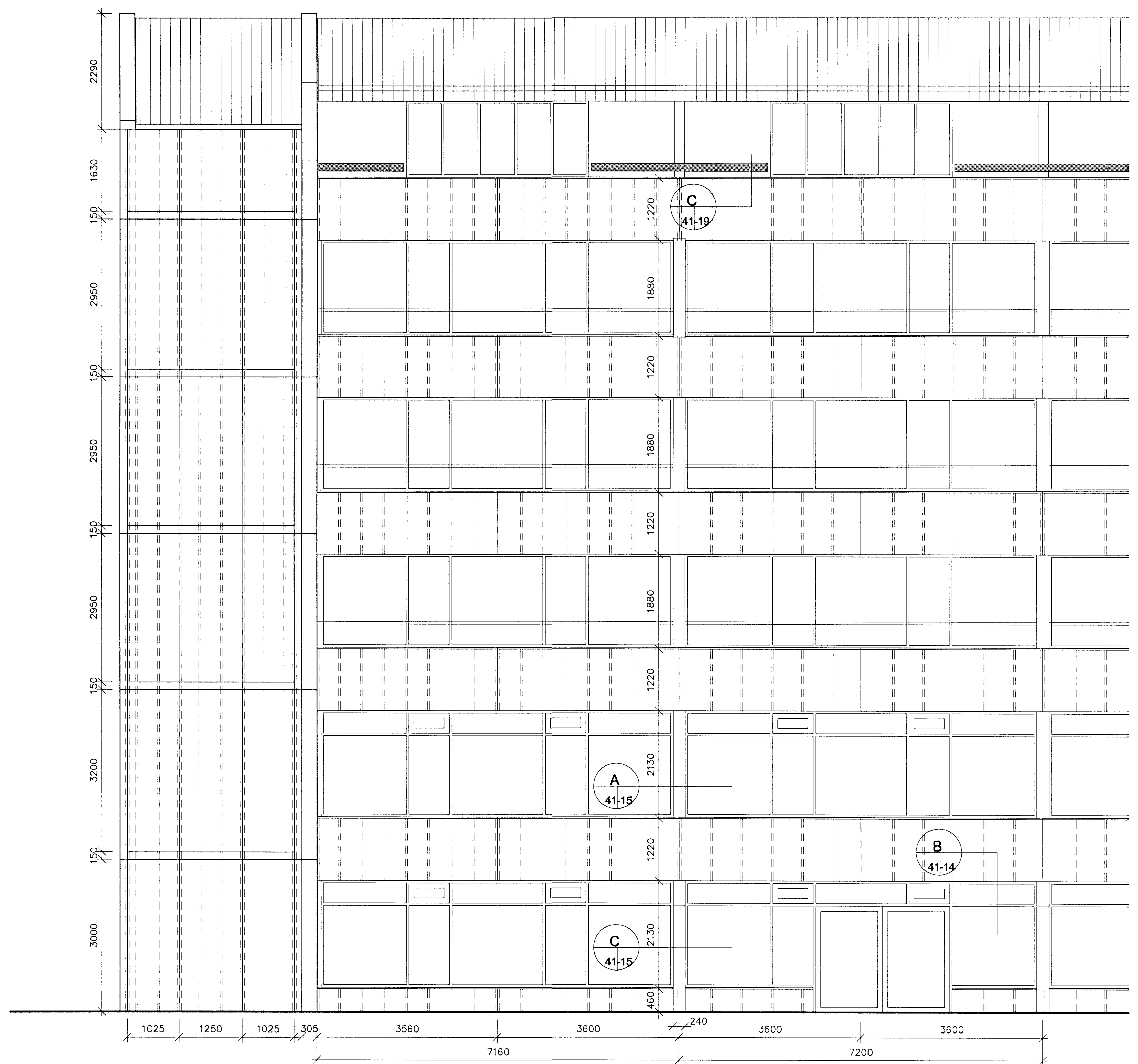
VESTURHLÍÐ NORÐURENDI A-ÁLMU 1:50
