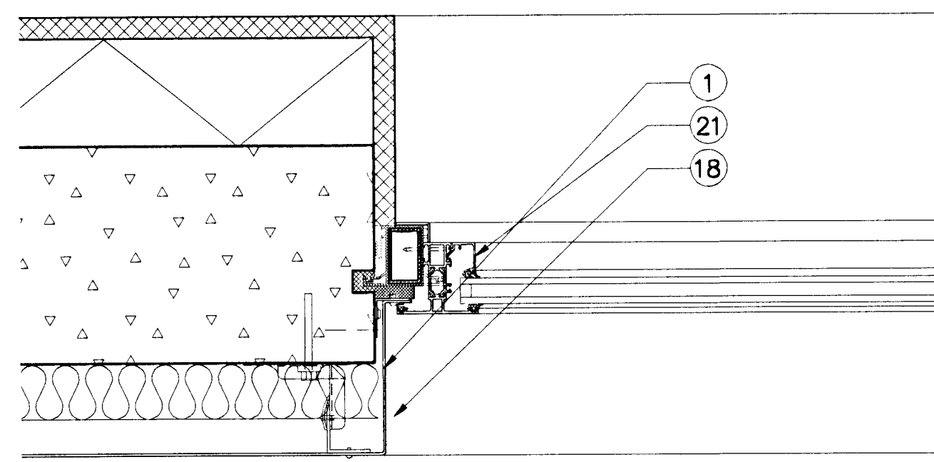
A 41-20 LÁRÉTT SNEIÐING VIÐ GLUGGA Á GAFLI B ÁLMU 1:5
