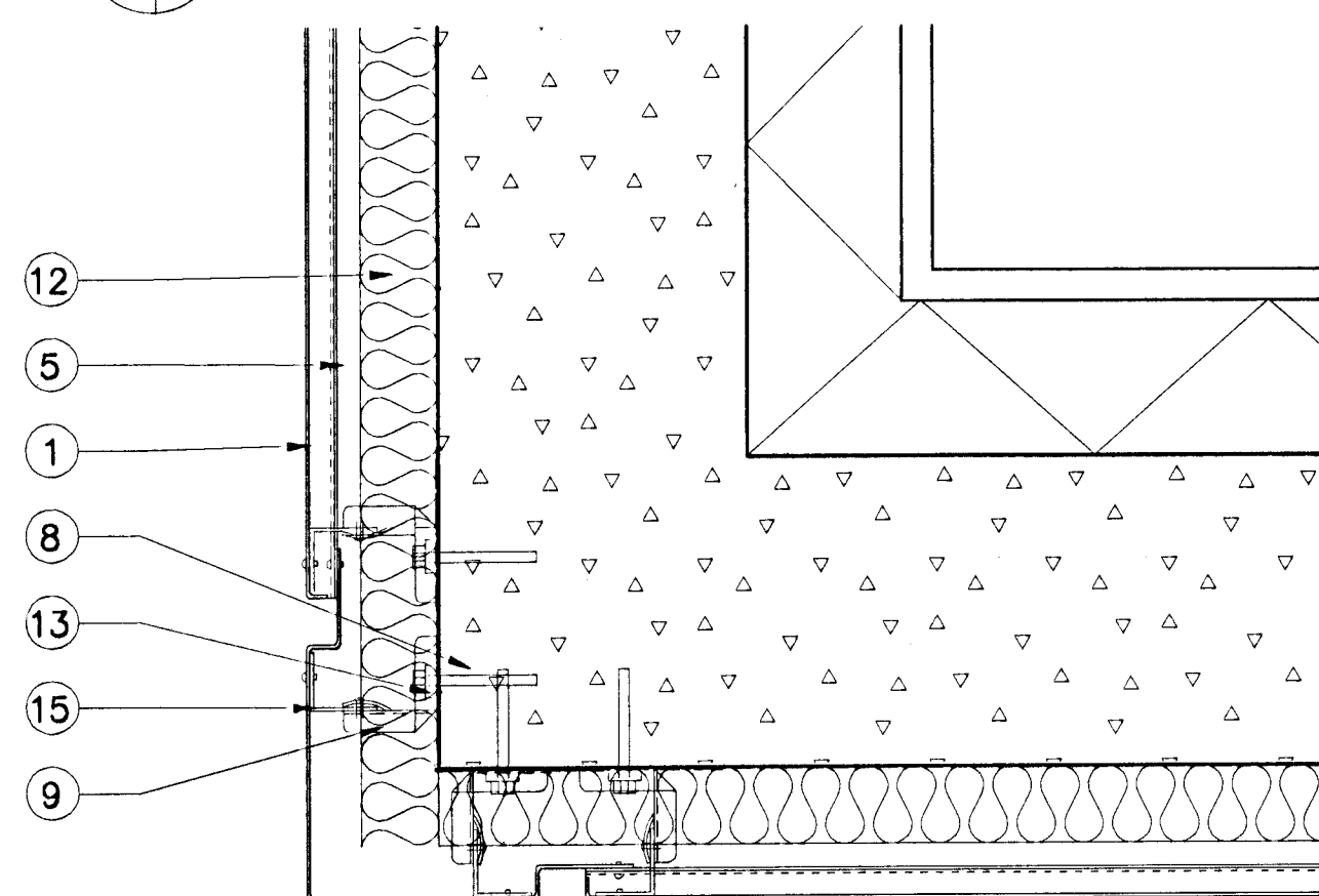
A 41-20 LÁRÉTT SNEIÐING Í INNHORN Á GAFLI A ÁLMU 1:5
