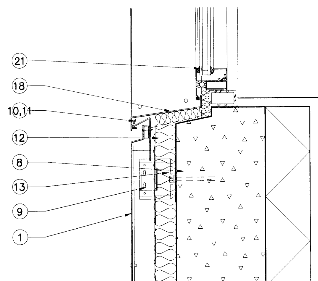
C 41-20 LÓDRÉTT SNEIÐING UNDIR GLUGGA Á GAFLI B ÁLMU 1:5
