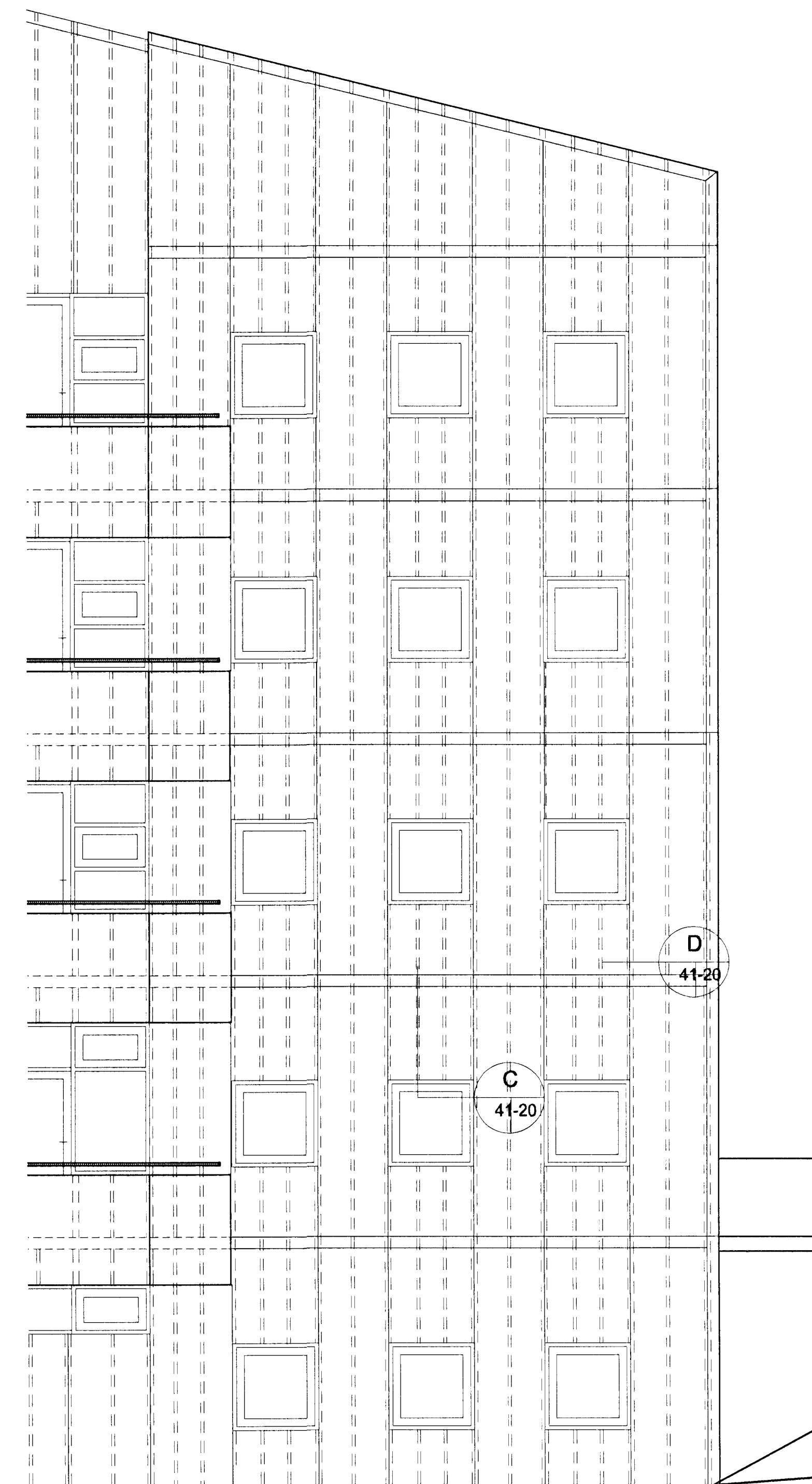
A 41-20 HLUTAÚTLIT GAFL B ÁLMU 1:50
