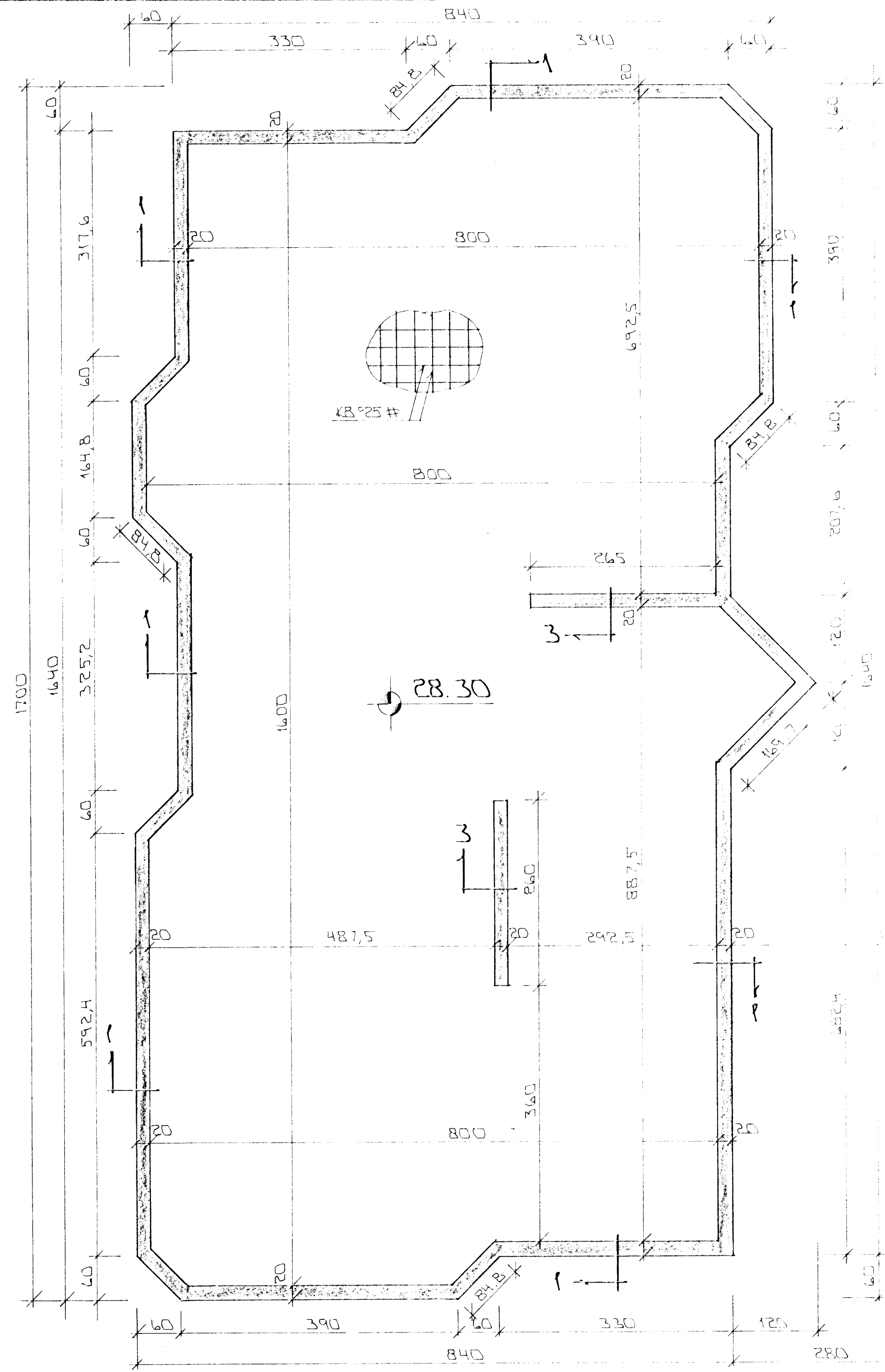
GRUNNMYND 1:50
