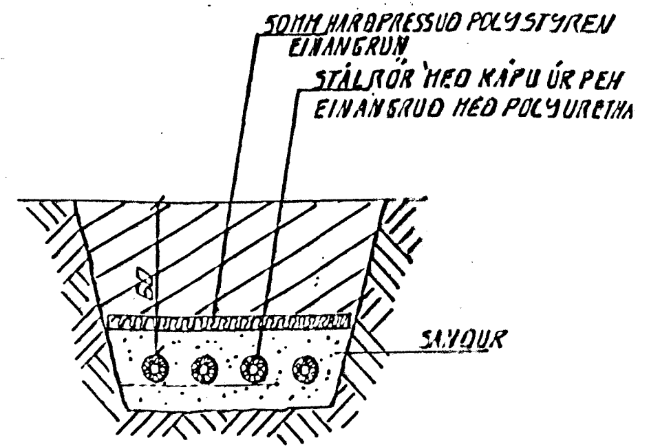
SNID 1:20 LAGNIR Í JÖRD
