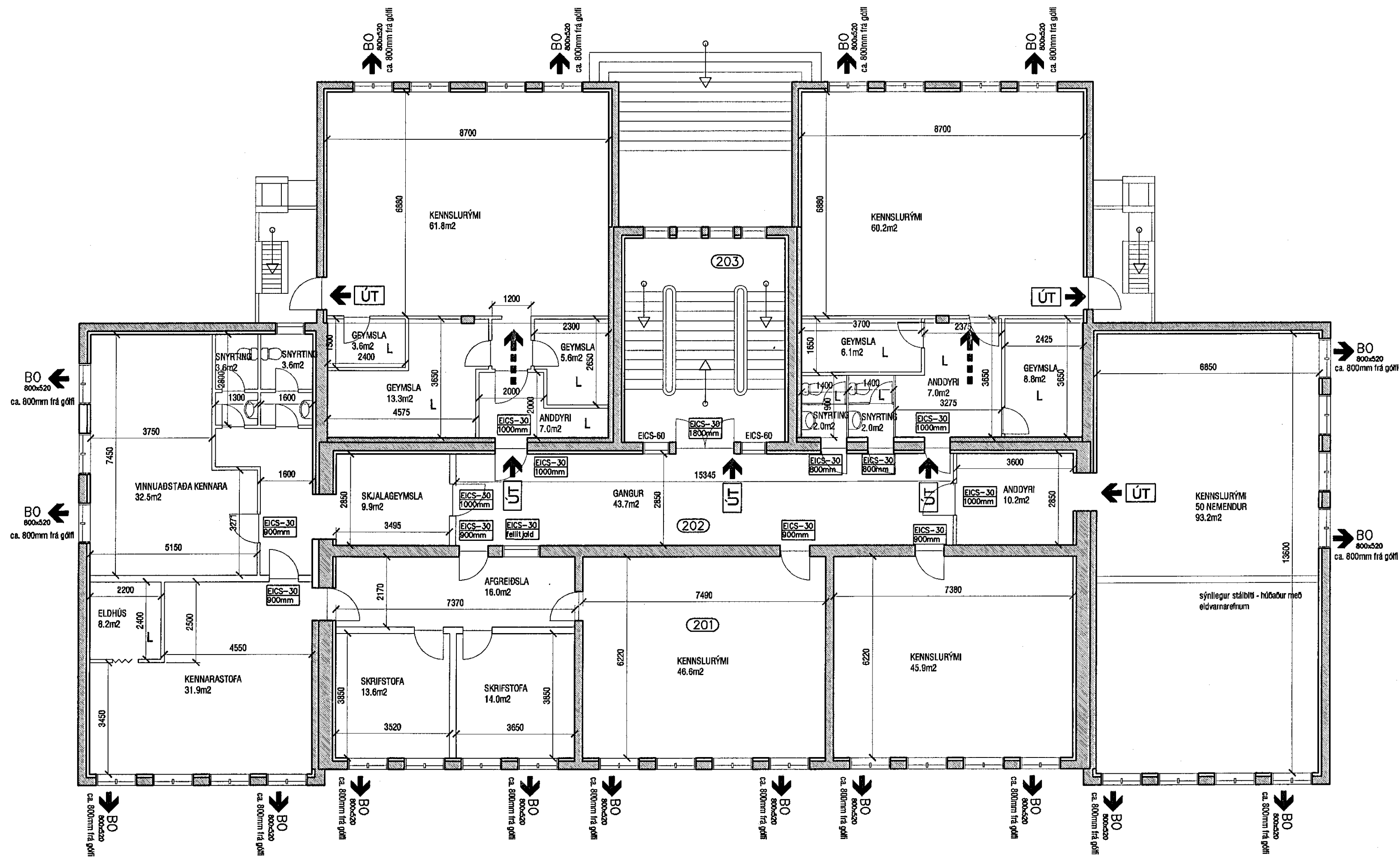
Grunnmynd 2. hæðar mkv. 1:100
