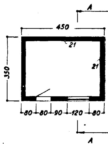
Grunnmynd
