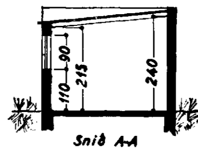
Snið A-A
