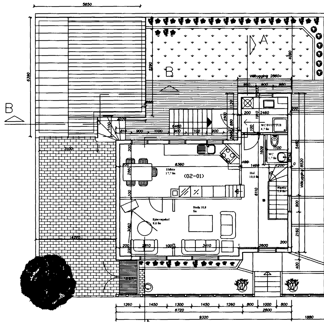
GRUNNMYND 1. HÆÐAR
