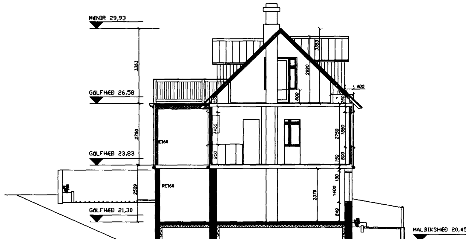
SNIÐ A-A
