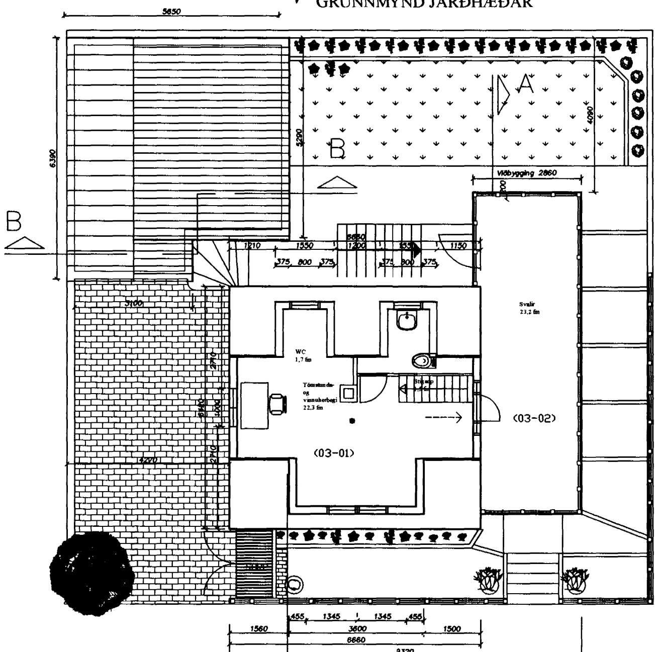
GRUNNMYND JARÐHÆÐAR
