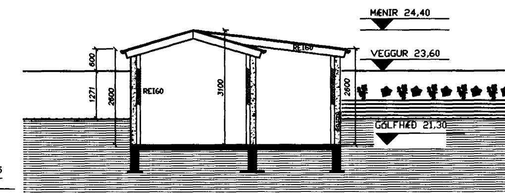
SNIÐ B-B
