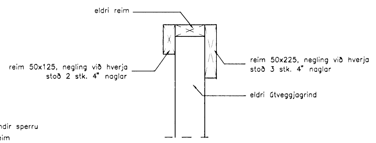
Snið 2-2 mkv. 1:10
