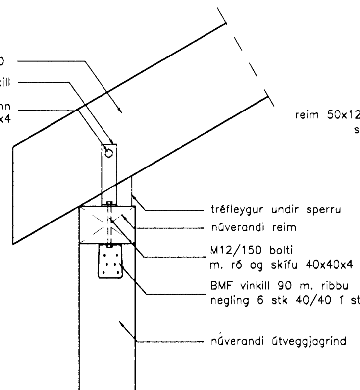
Snið 1-1 mkv. 1:10
