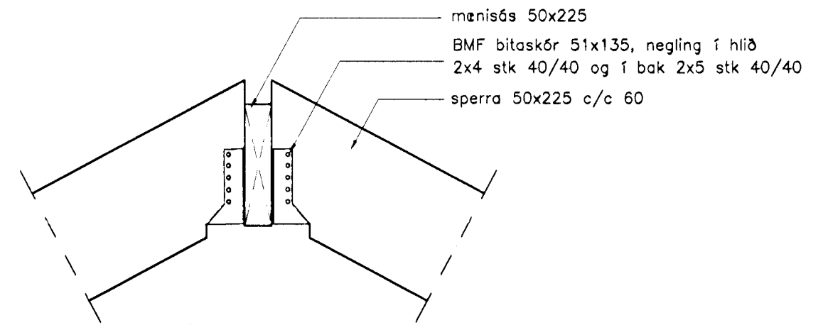
Snið 4-4 Mkv. 1 : 10
