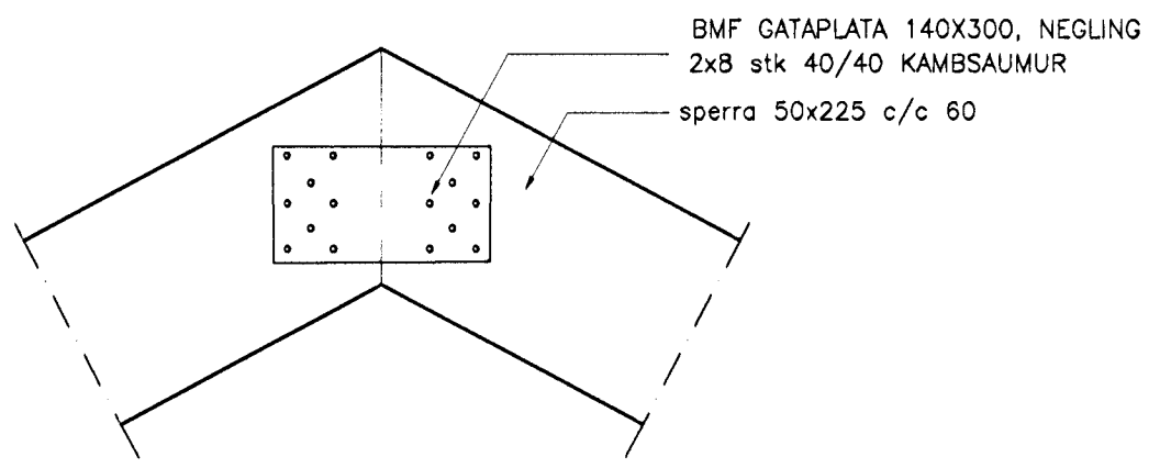
Snið 3-3 Mkv. 1 : 10
