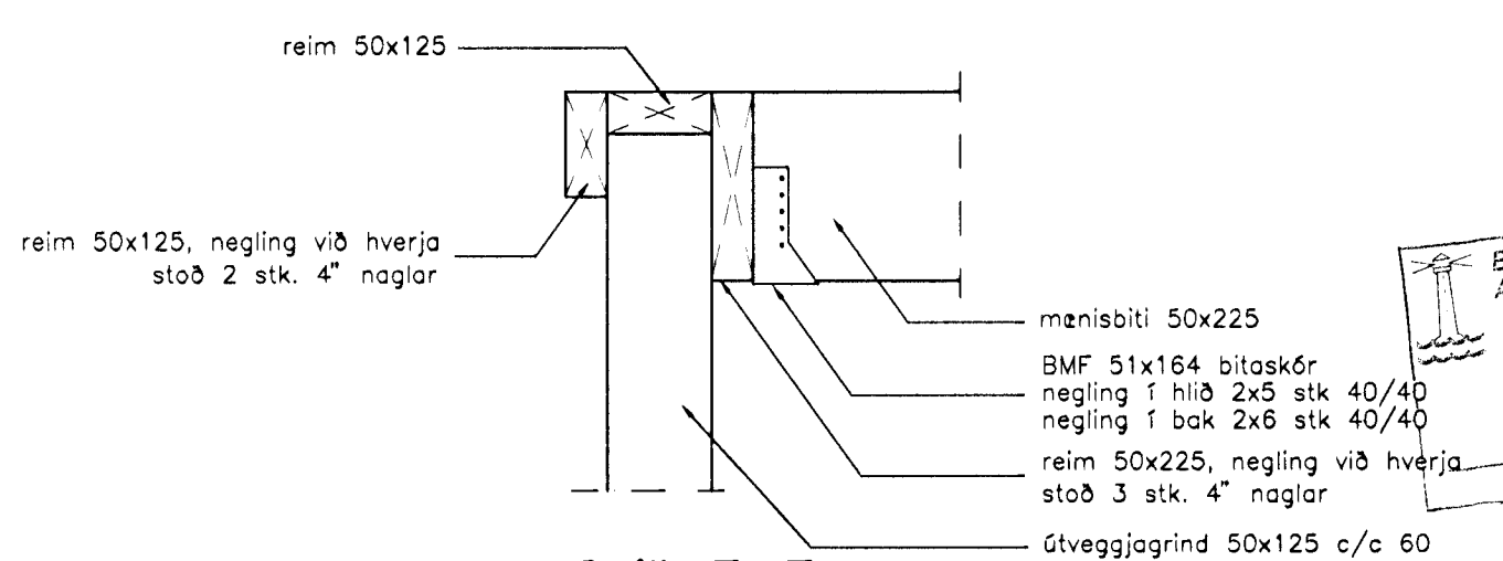
Snið 7-7 mkv. 1:10
