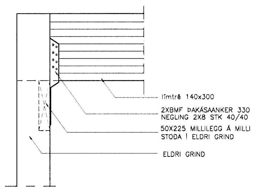
Snið 6-6 mkv. 1:10
