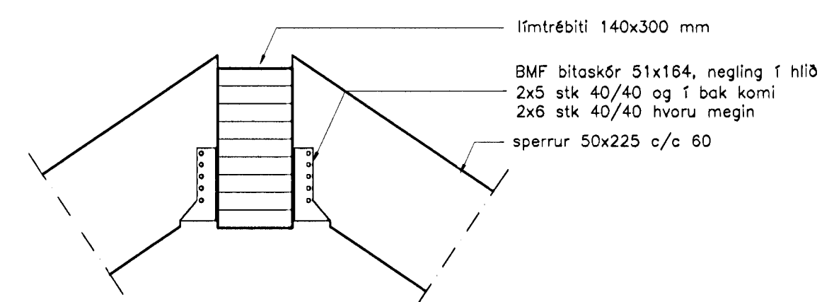
Snið 5-5 mkv. 1:10
