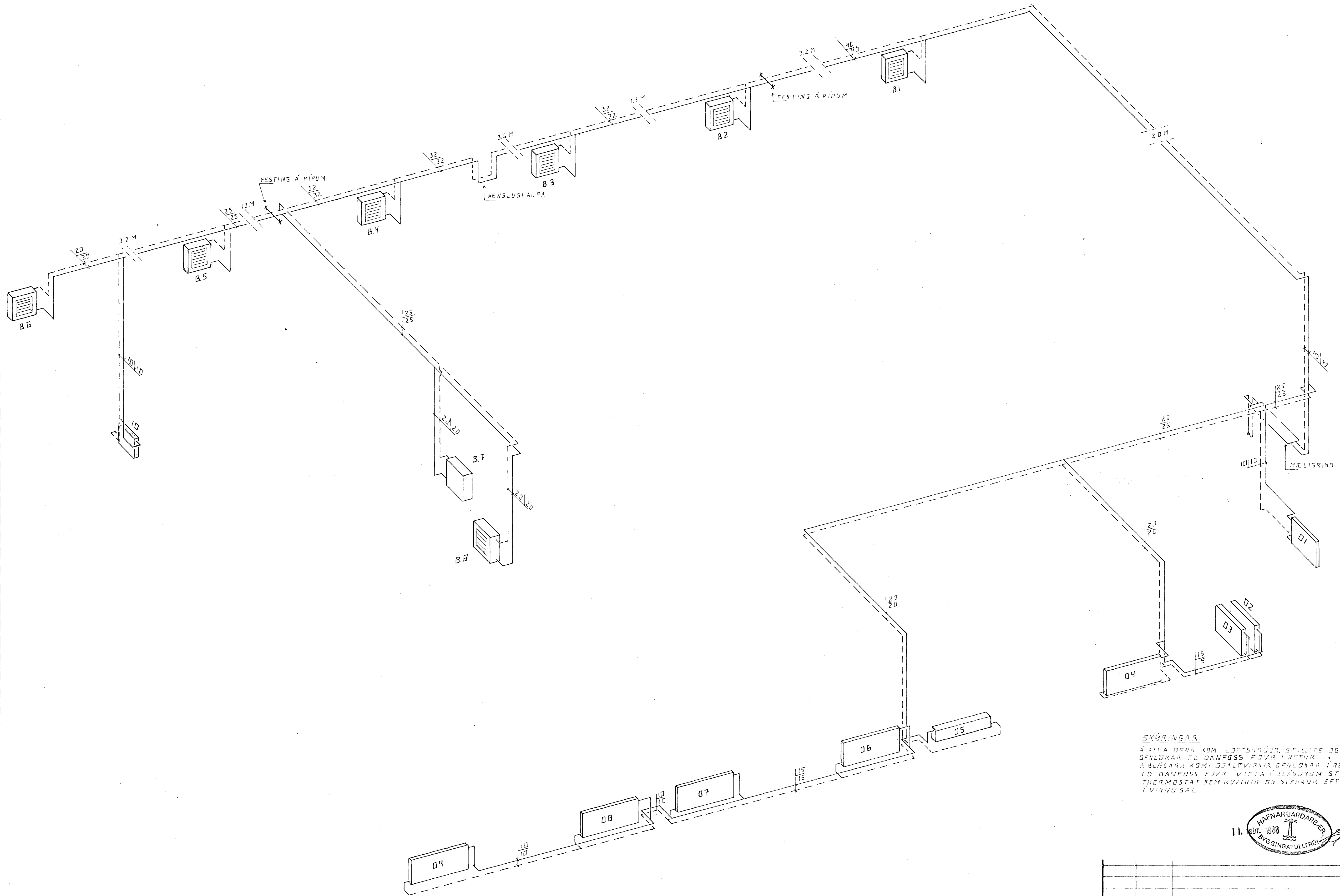
RÚMMYND 1:50
