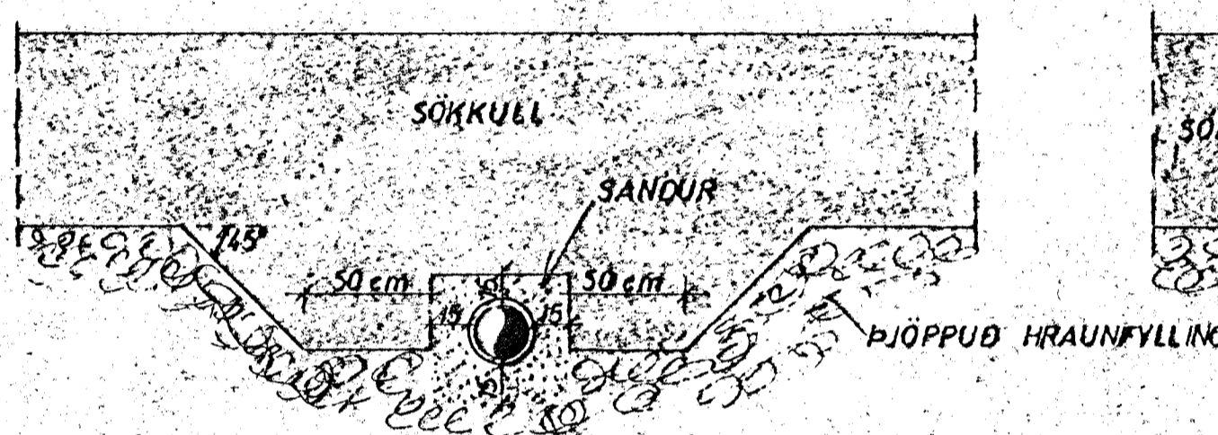
GRAFID SKAL FYRIR LÖGNUM UNDIR SÖKKLUM, AÐUR EN ÞEIR ERU STEYPTIR
