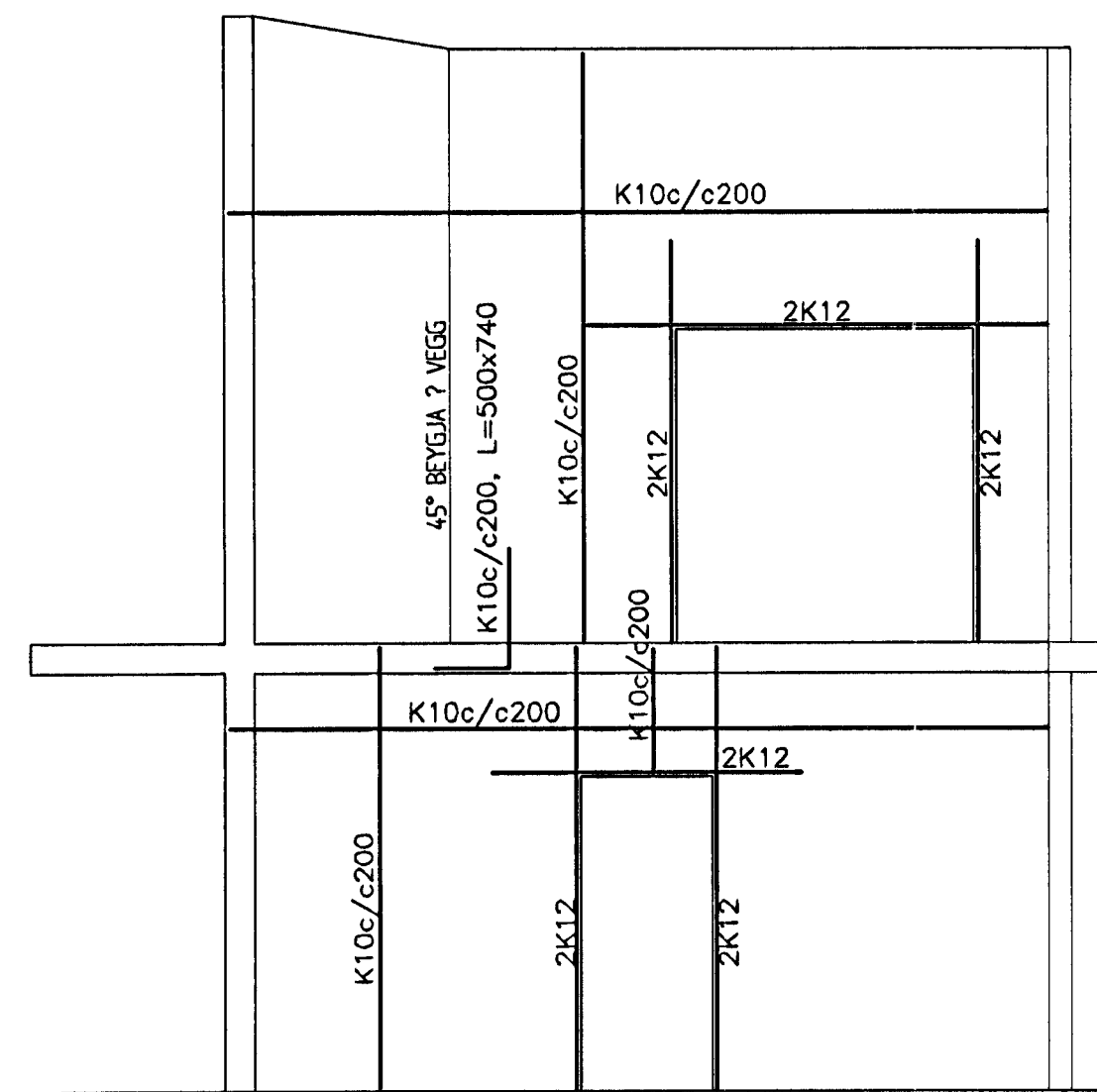
INNVEGGUR C 1:50
