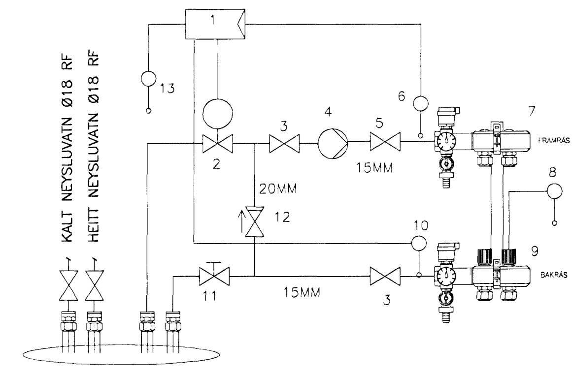
Ø22 PEX-RÖR Í Ø40 4.STK. IDRÁTTARÖRI FRÁ TÆKNIRYMI
