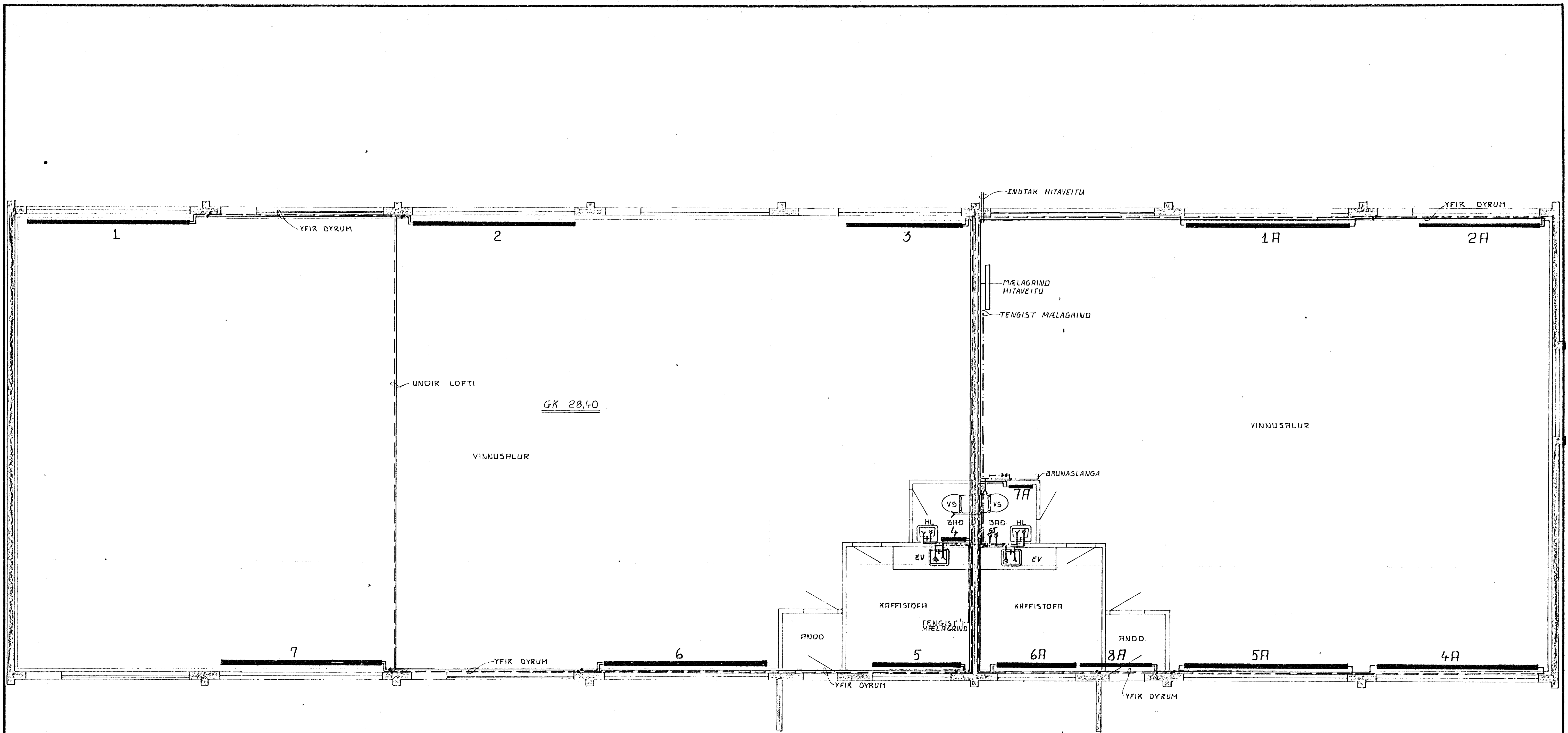
GRUNNMYND 1:50
