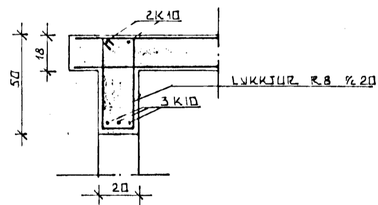
SNIEDI BITA YFIR GLUGGA OG HURÐ 1:20
