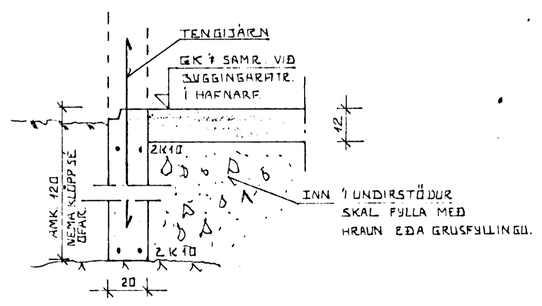
KENNISNIÐ Í UNDIRSTÖÐUR 1:20.
