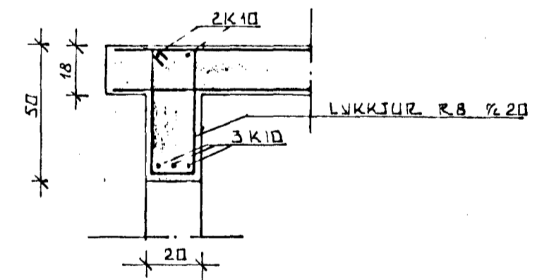
SNÍÐI ÞITA YFIR GLUGGA OG HURÐ 1:20
