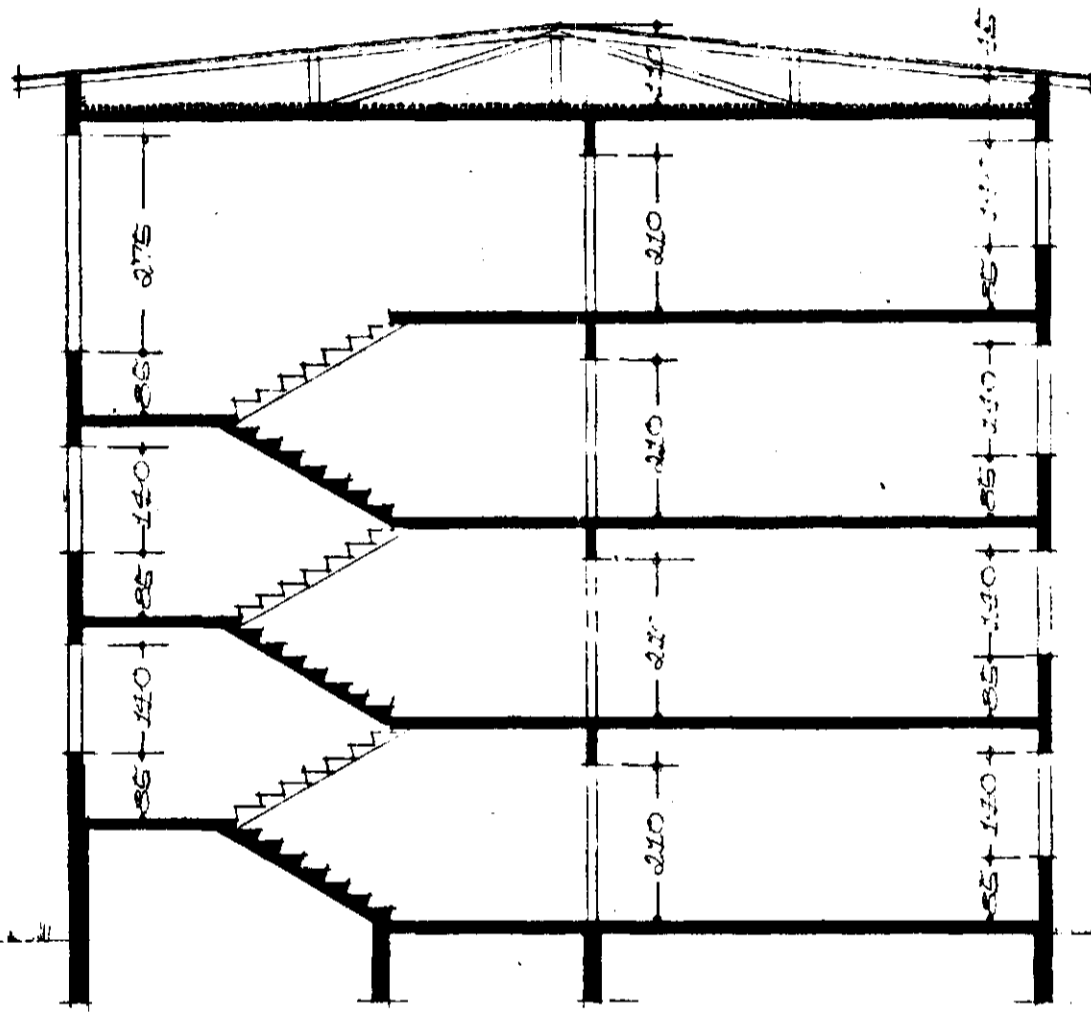
STURÐUR B-B
