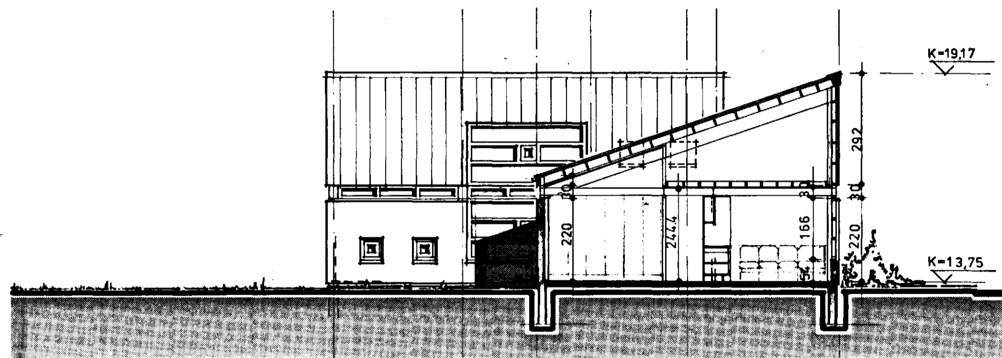
sneiding a-a
