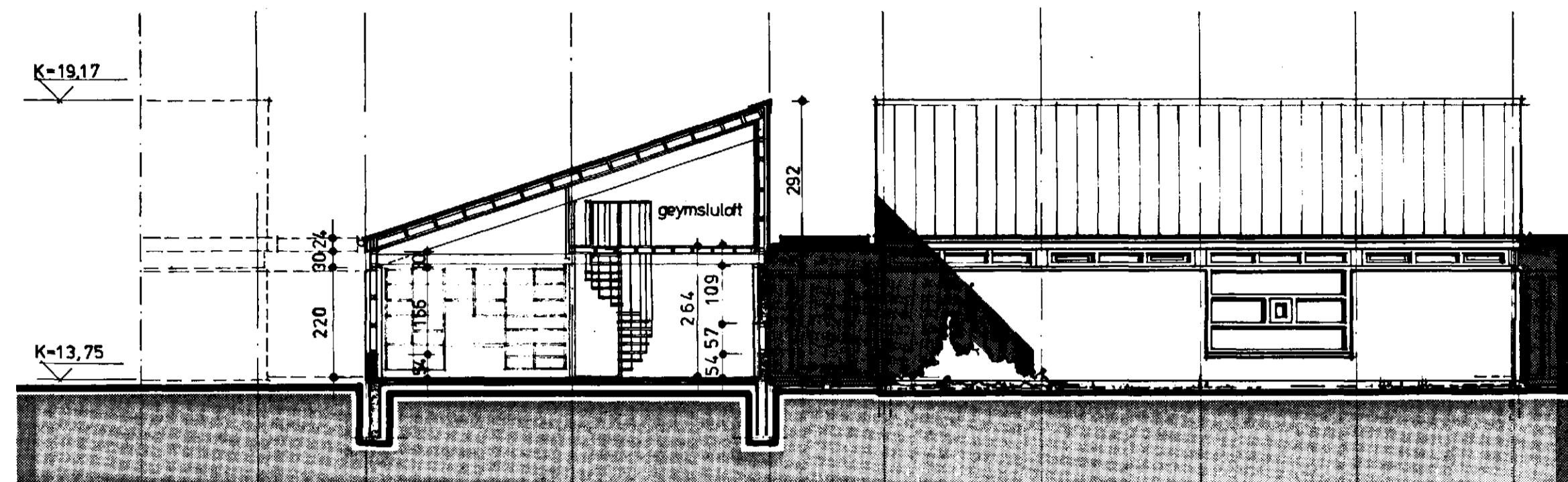
sneiding b-b
