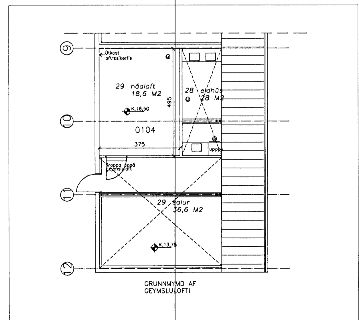
GRUNNMYND GEYMSLULOFTS
