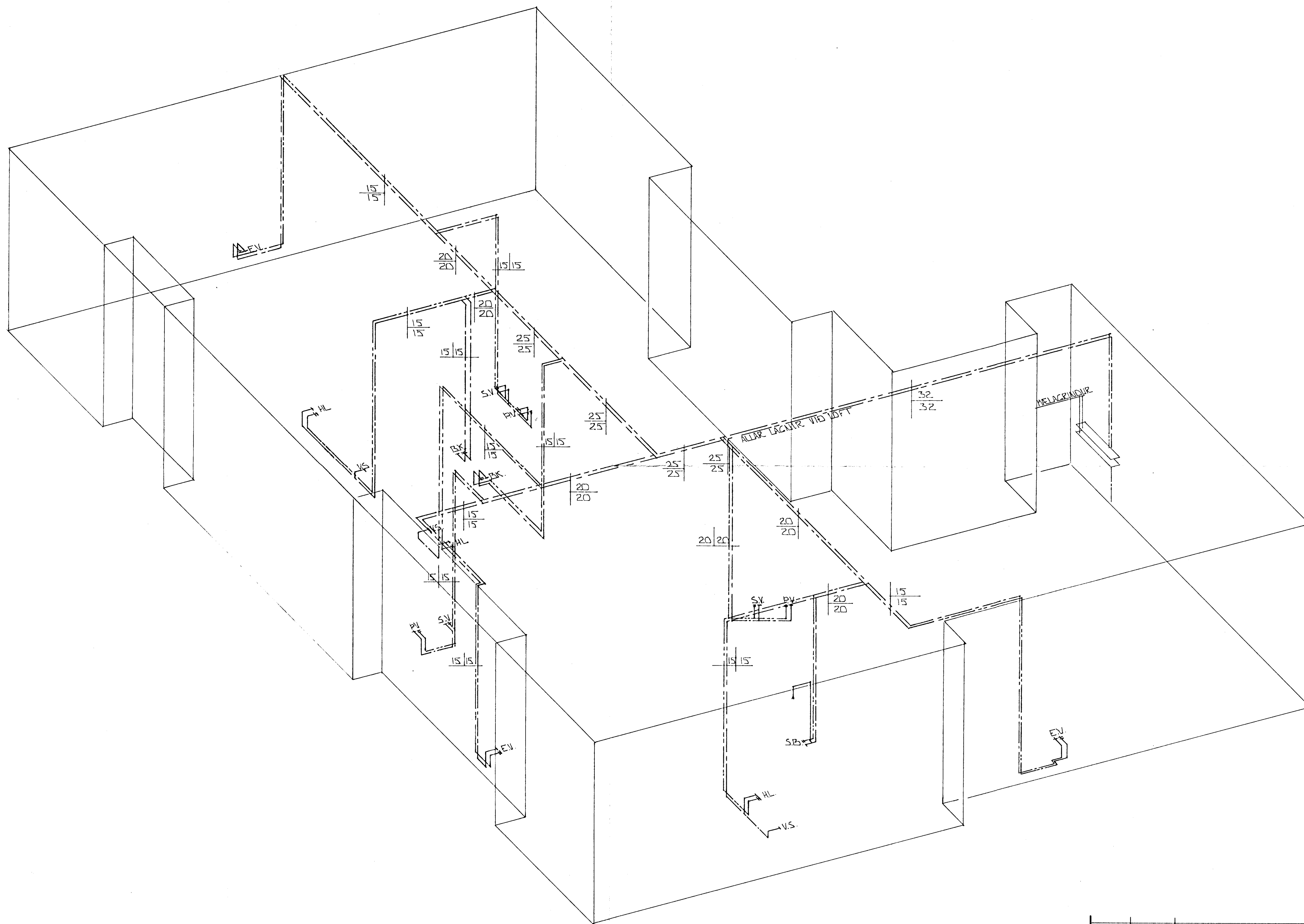
RÚMMIND VATNSLAGNA • 1:50
