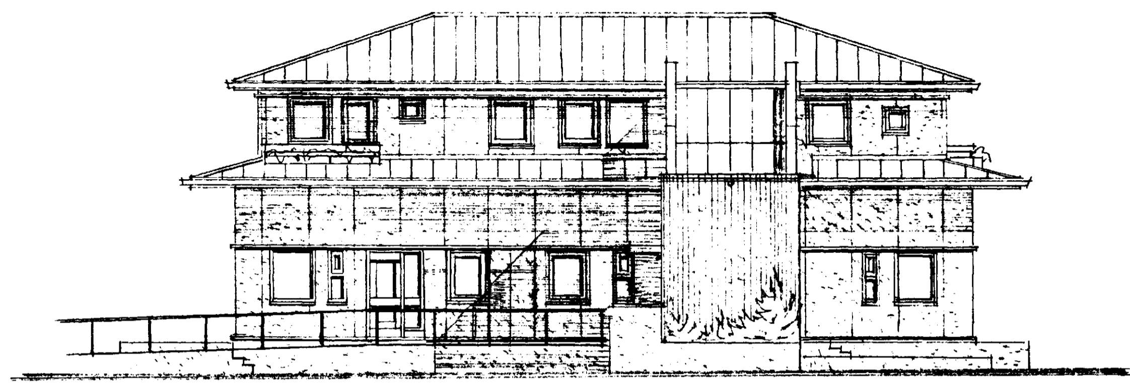
NORÐAUSTUR M. 1:100
