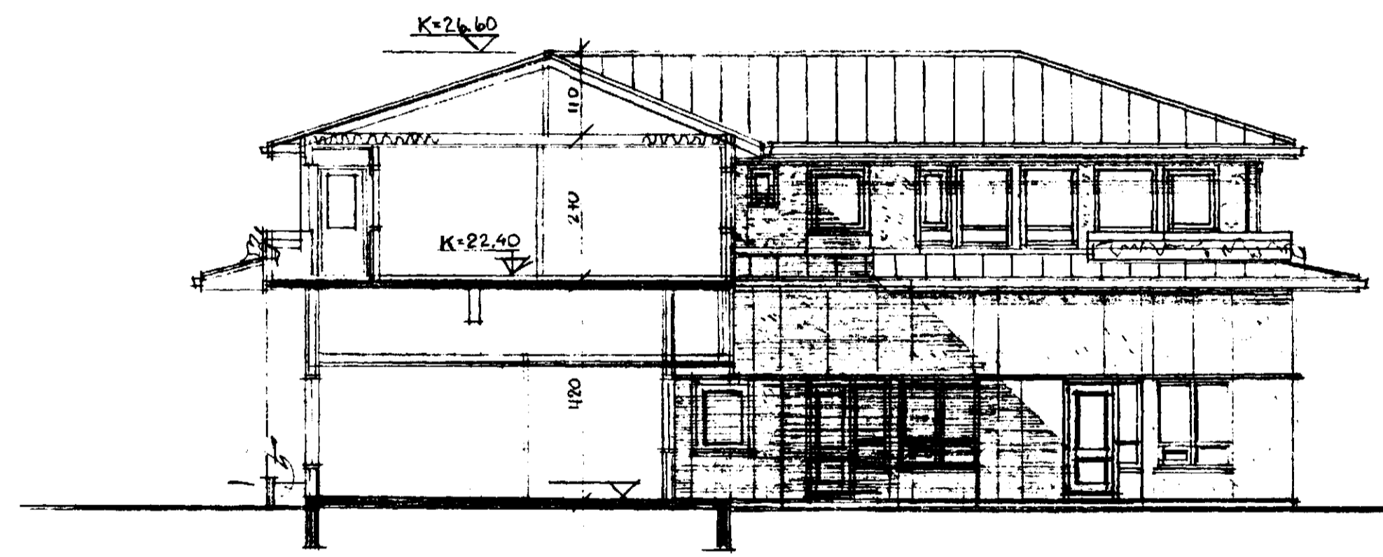
SUÐVESTUR M. 1:100
