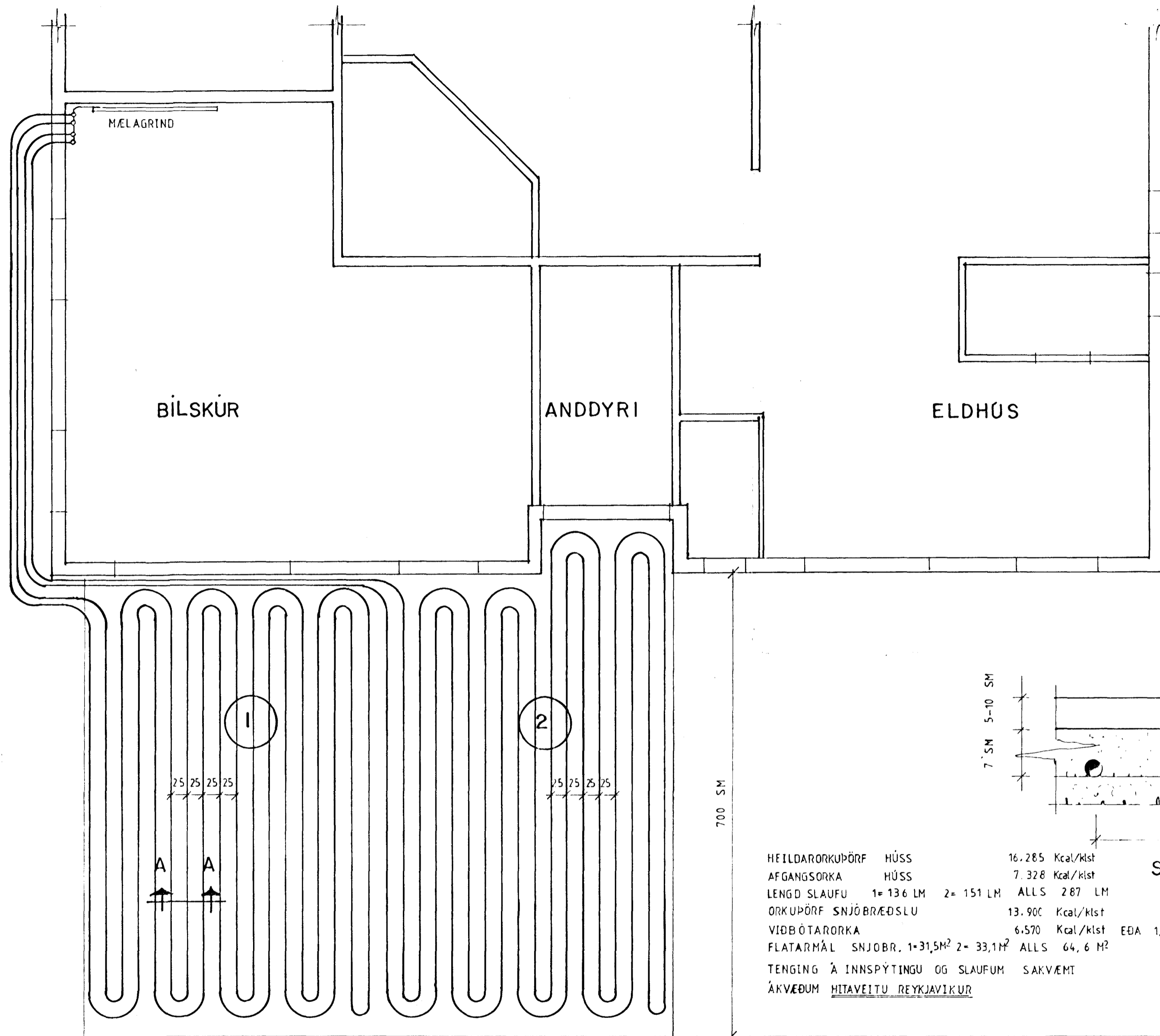
GRUNNMYND 1:50
