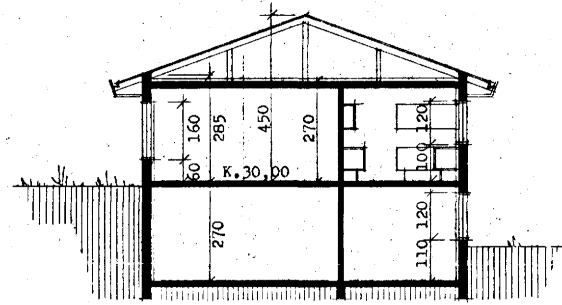
skurður A-A
