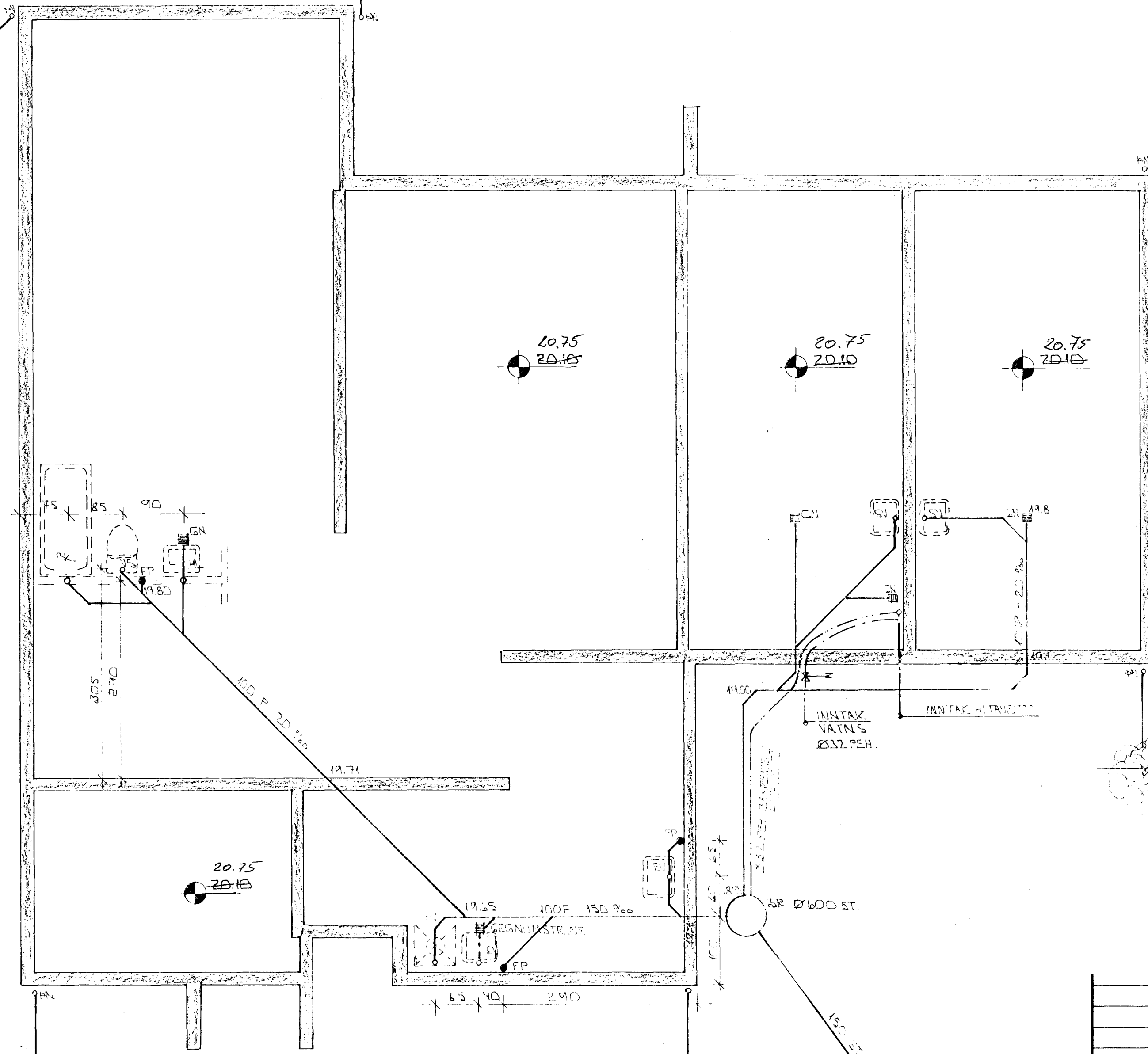
GRUNNMYND · 1:50
