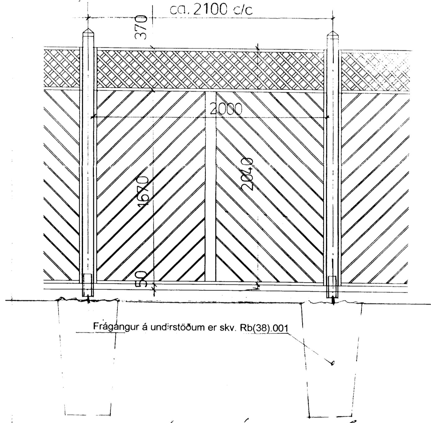
Útlit af dæmigerðum skjólveggis-panil Mkv. 1:20
