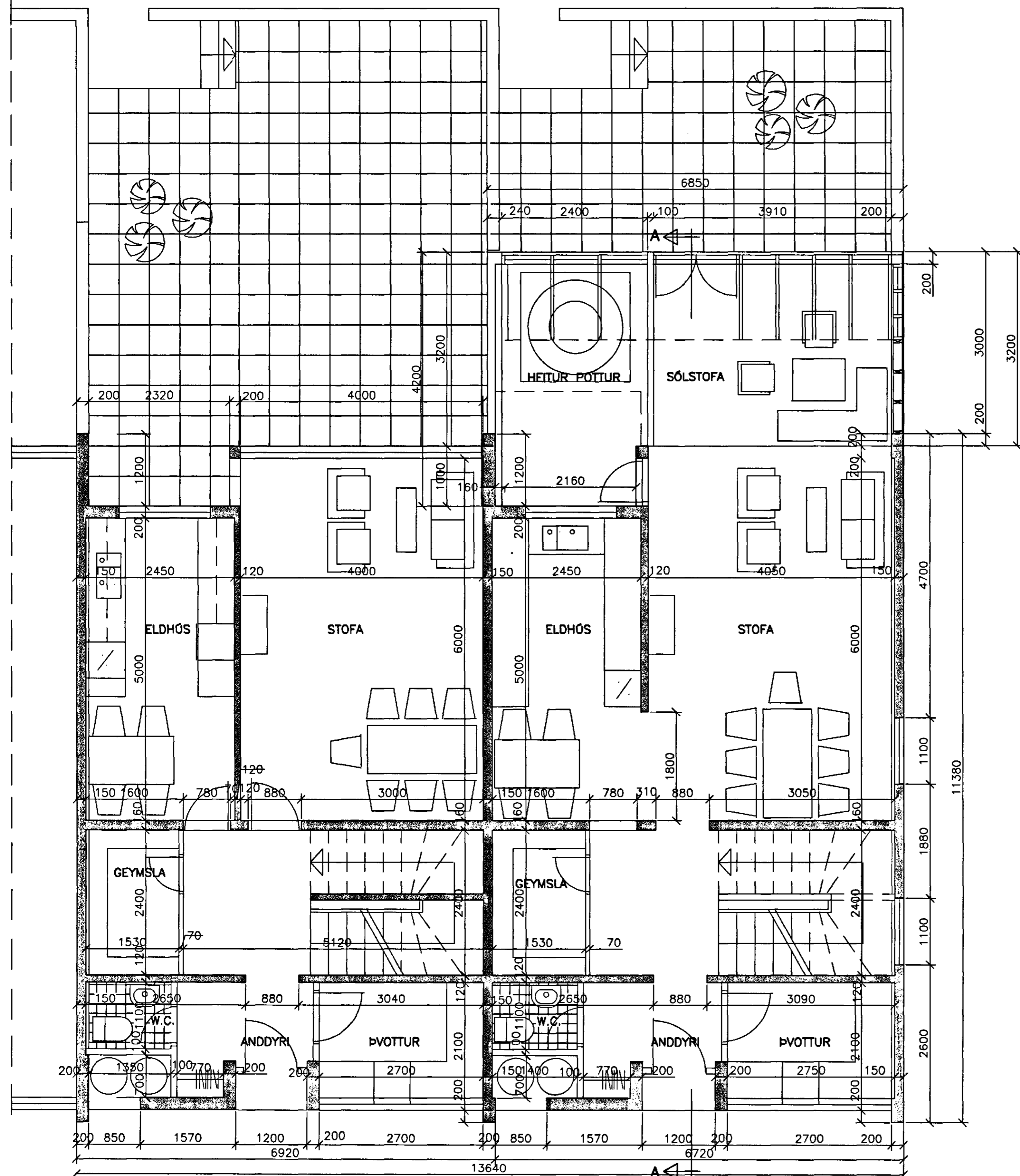
GRUNNMYND 1.HÆÐAR
