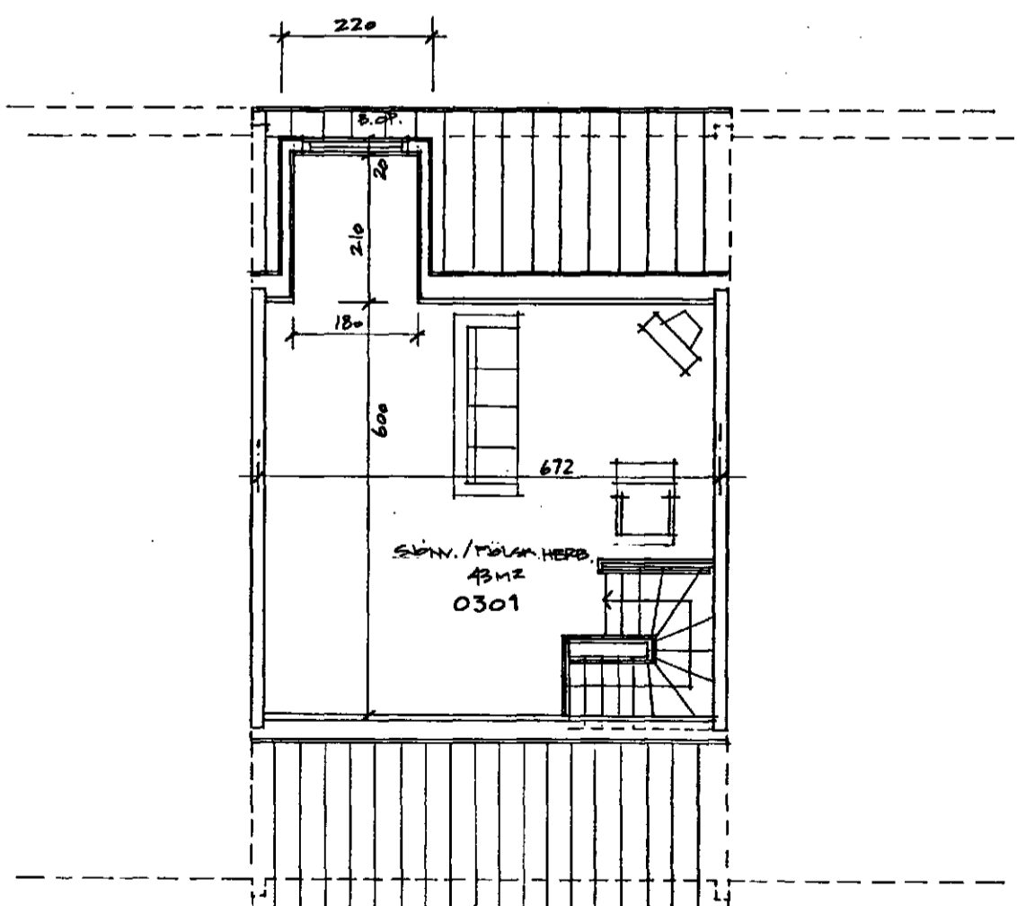
GRUNNMYND RISHÆÐ, 1:100
