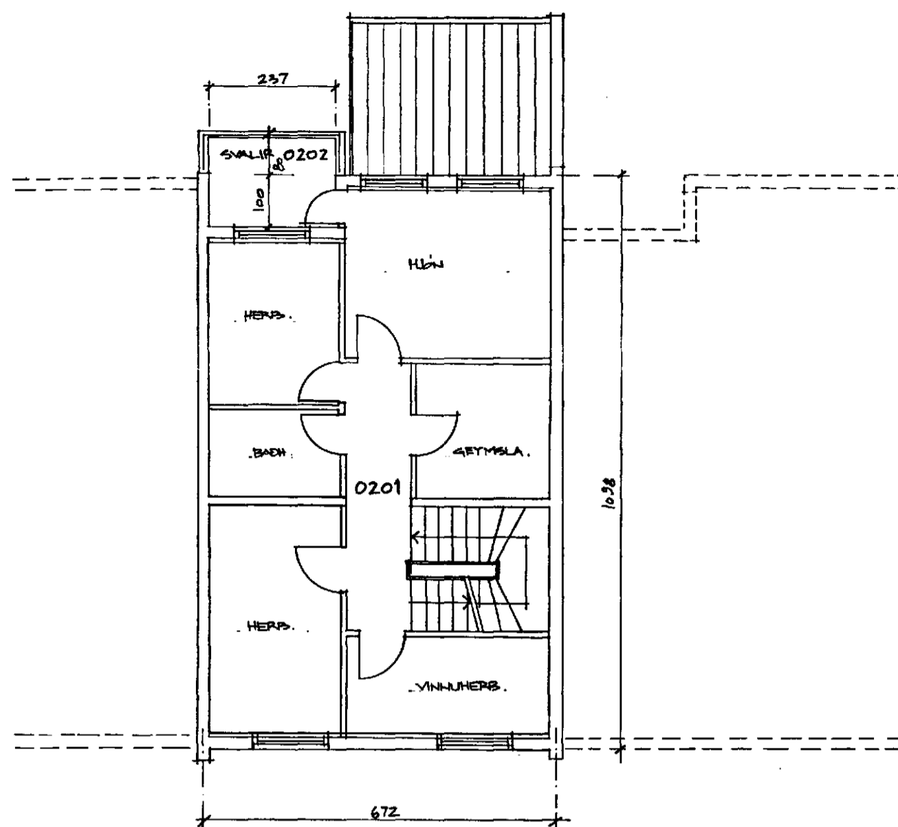
GRUNNMYND 2. HÆÐ, 1:100
