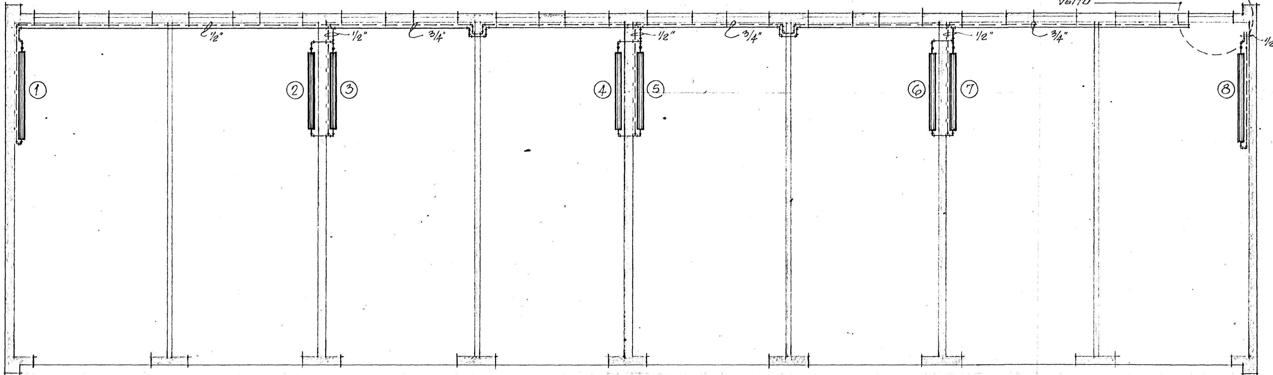
GRUNNMYND MKV = 1:50
