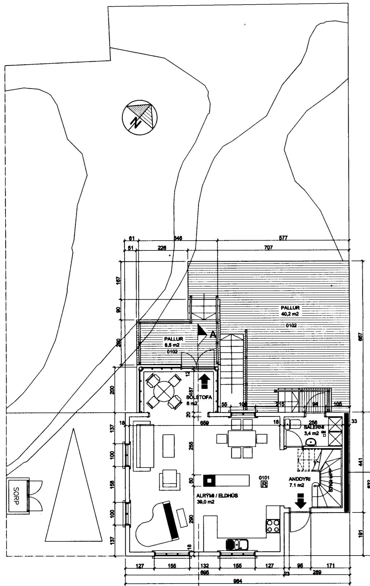
GRUNNMYND 1. HÆÐAR 1:100
