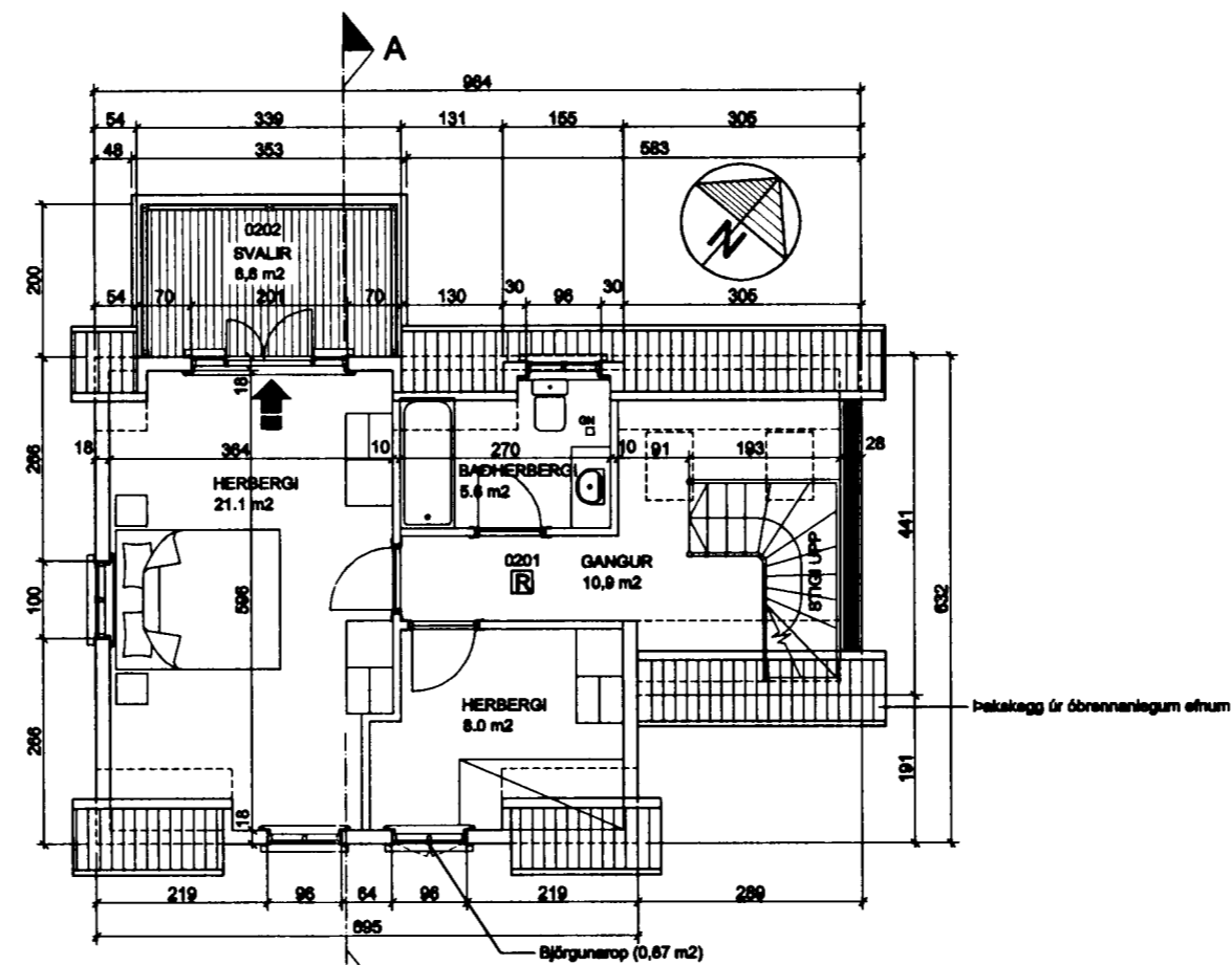
GRUNNMYND RISHÆÐAR 1:100
