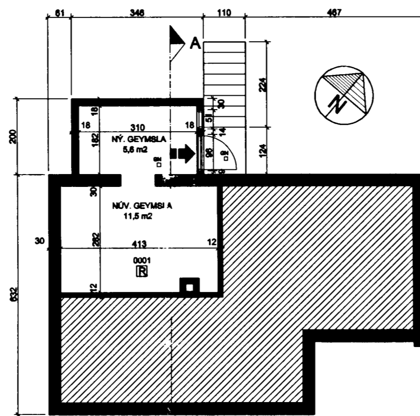
GRUNNMYND RISHÆÐAR 1:100
