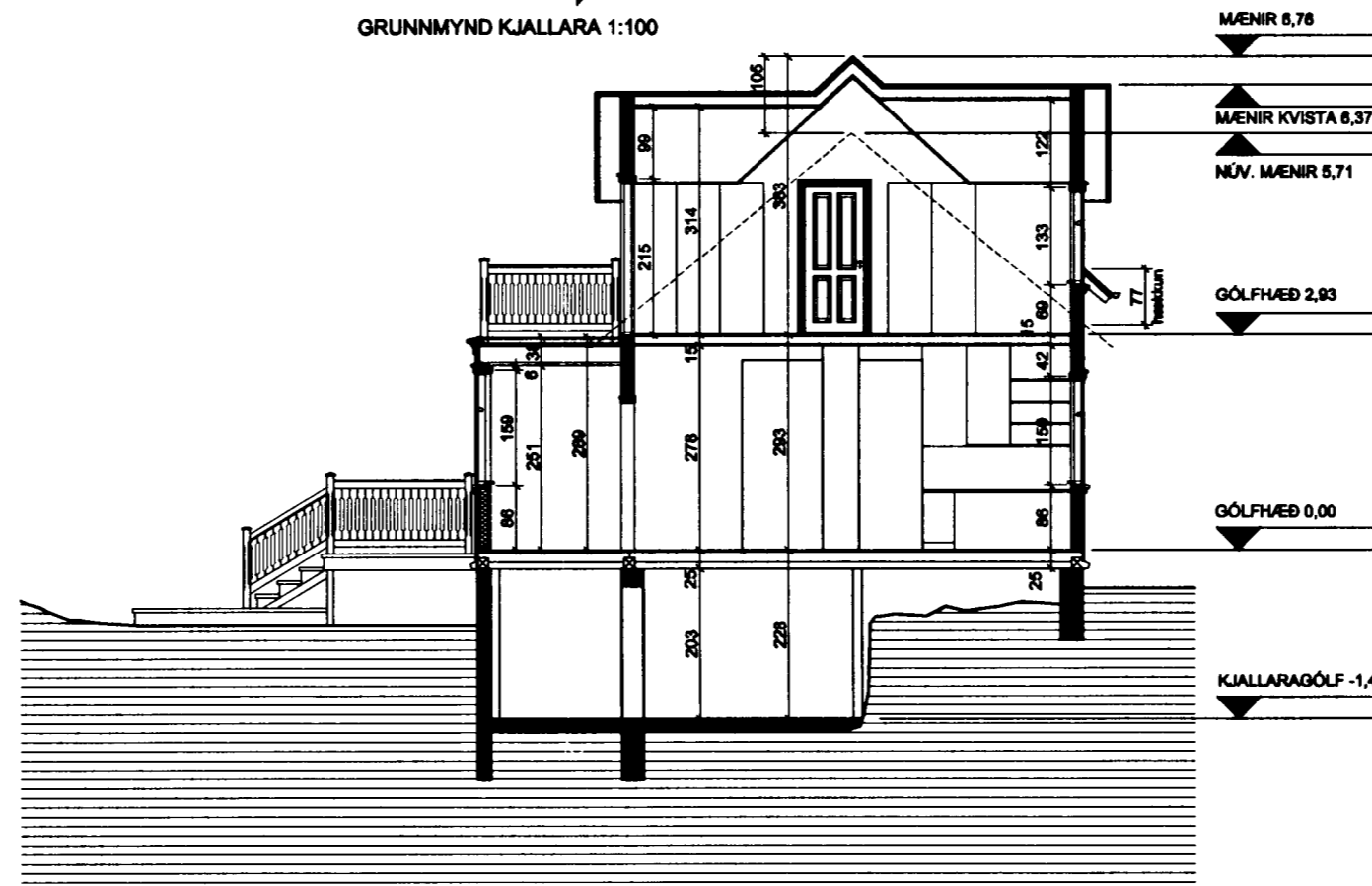
DVERSKURÐUR 1:100
