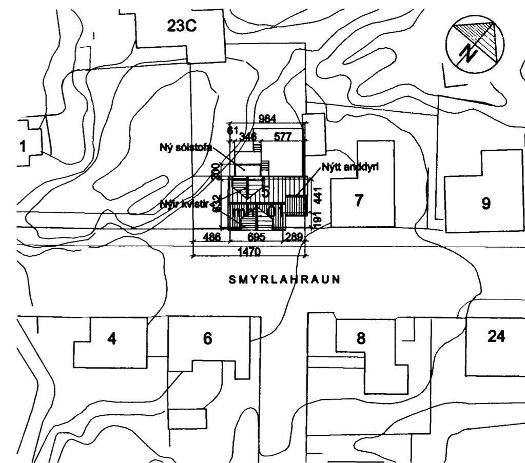
AFSTÖÐUMYND 1:500
