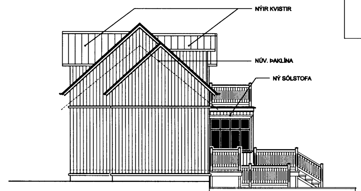
ÚTLIT NORÐAUSTURGAFL 1:100
