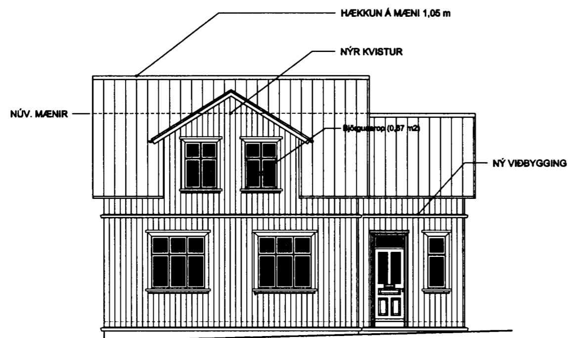
ÚTLIT SUBAUSTURHLÍÐ 1:100
