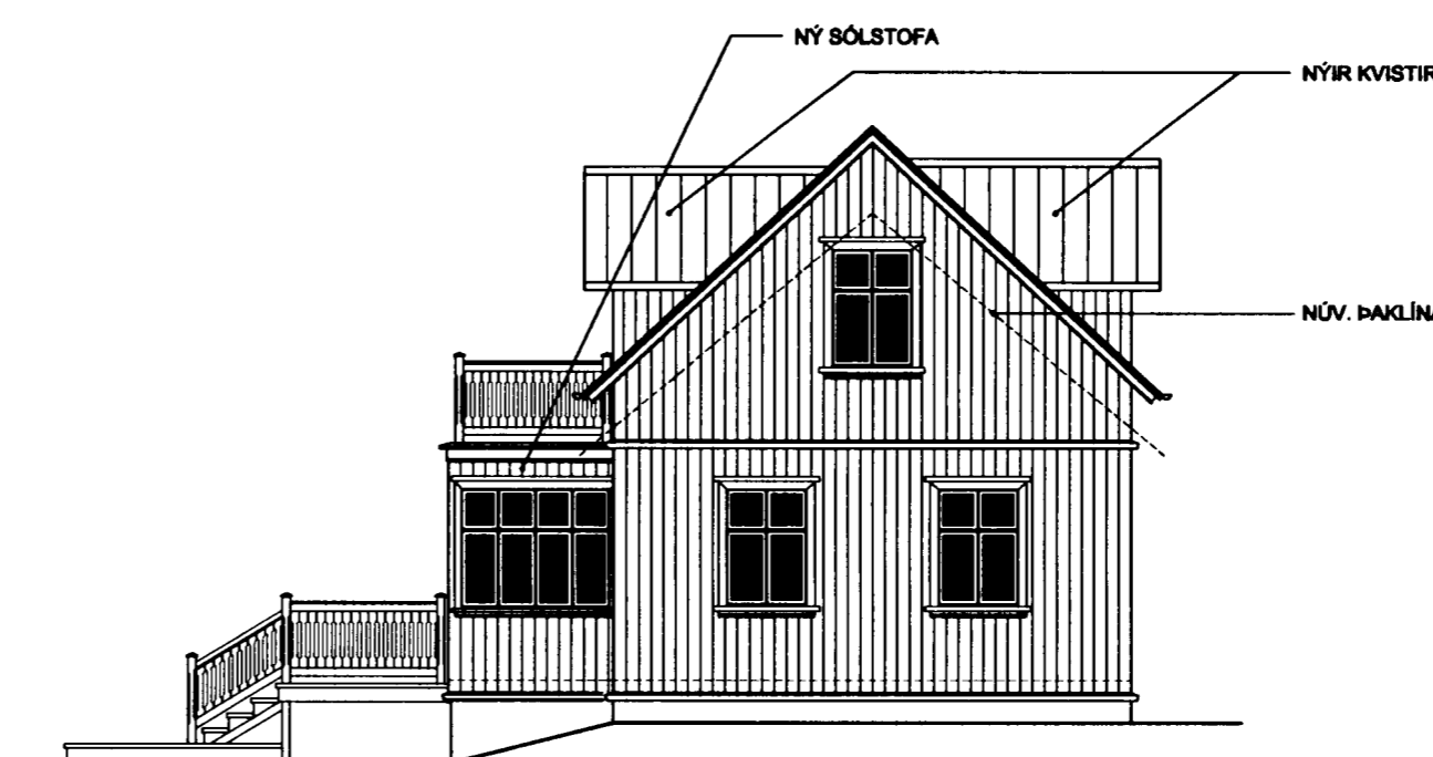
ÚTLIT SUÐVESTURGAFL 1:100
