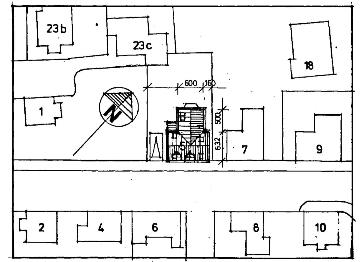
AFSTÖÐUMYND 1:100
