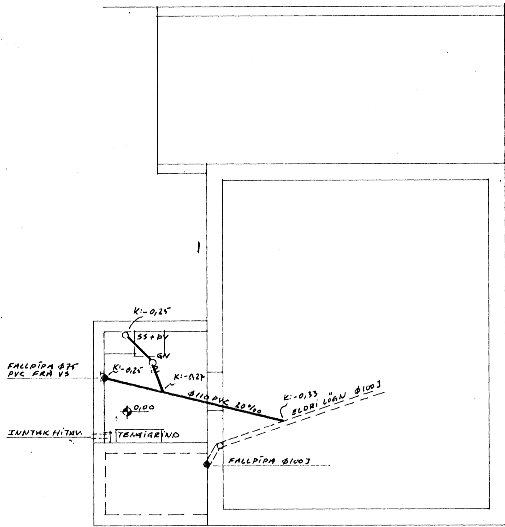
GRUNNMYND KTALLARA 1:50
