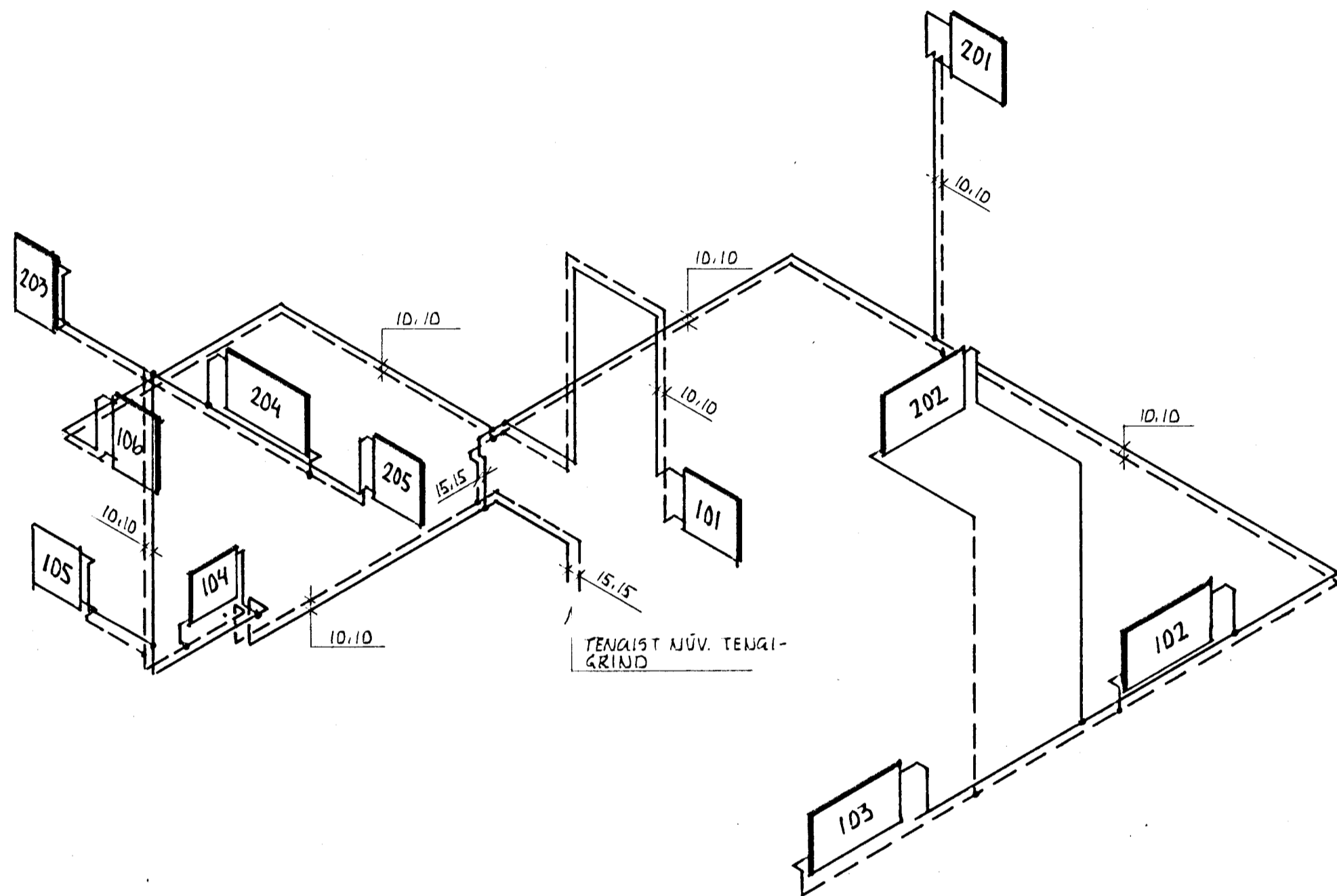
RÚMMYND HITAKERFIS 1:50
