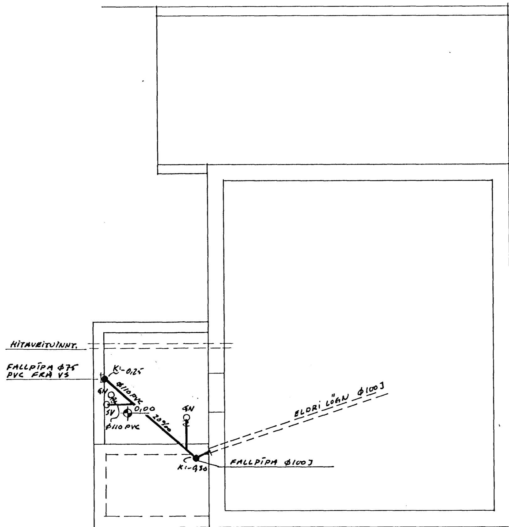
GRUNNMÝND KJALLARA 1:50
