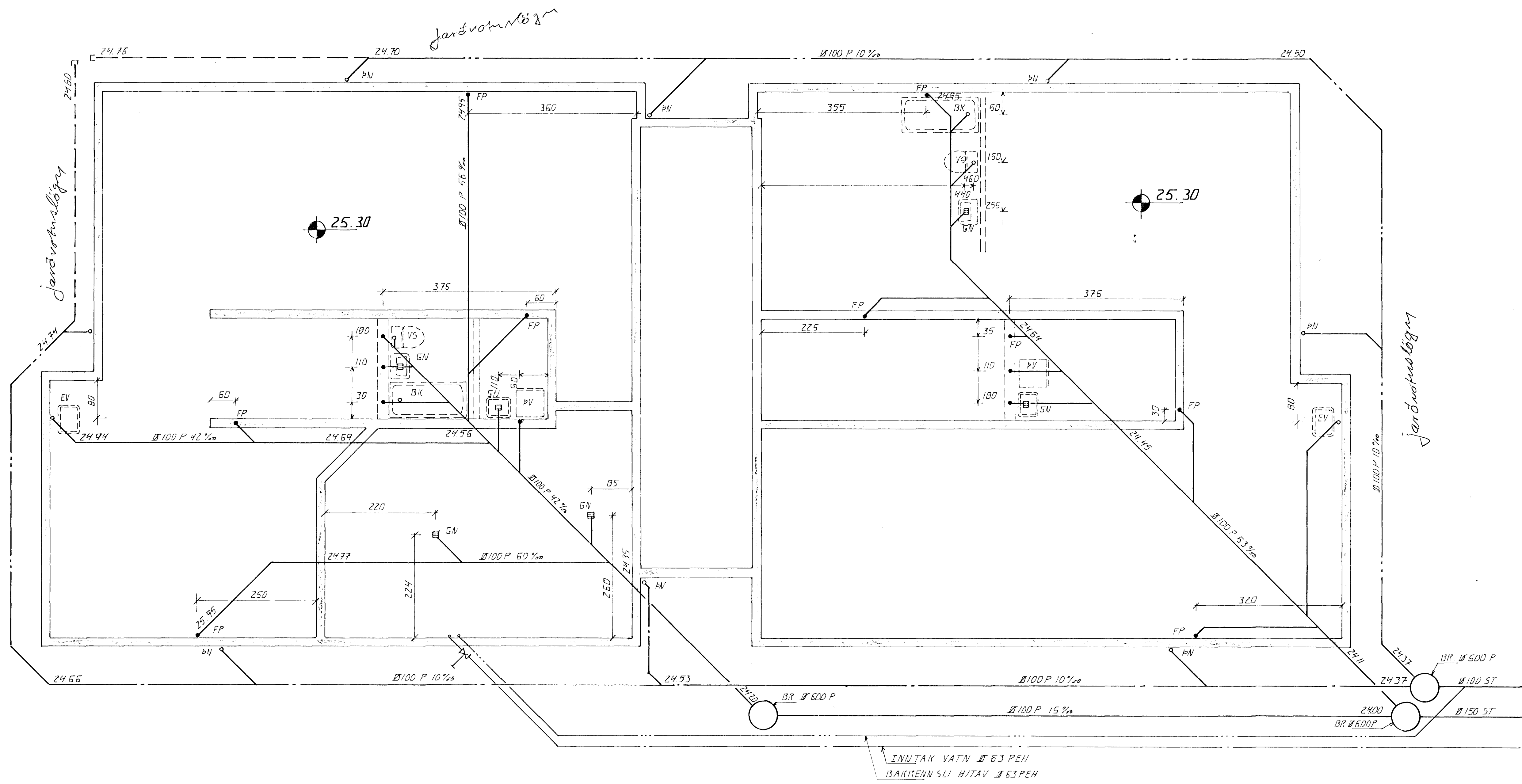
GRUNNMYND . 1:50
