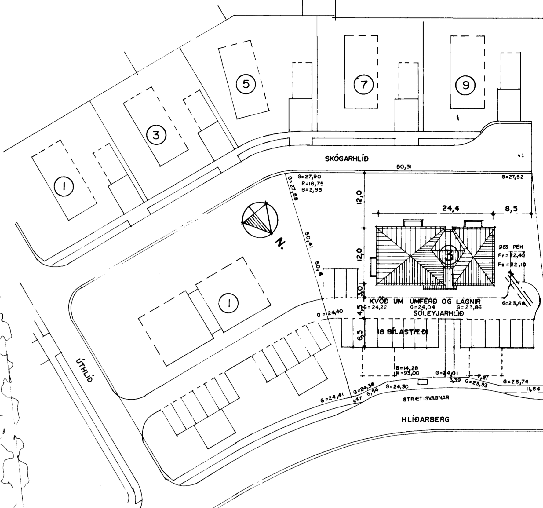
AFSTÖÐUMYND MKV. 1:500
