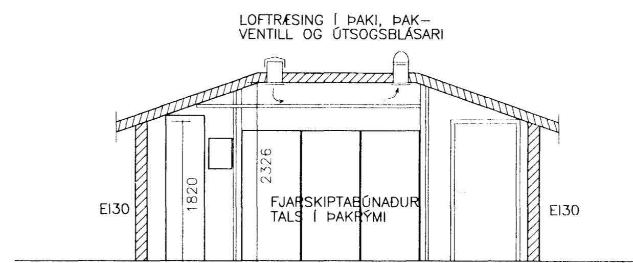
SNID 1-1 TÆKJAHERBERGI 1:50
