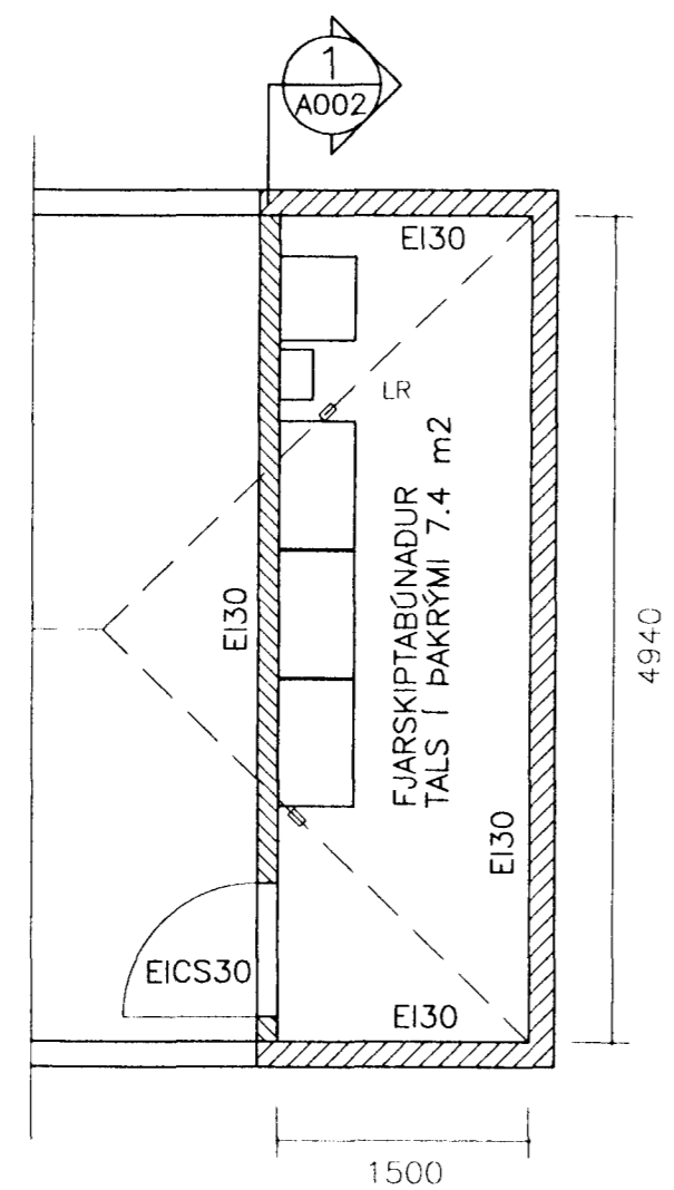
GRUNNMYND TÆKJAHERBERGI 1:50
