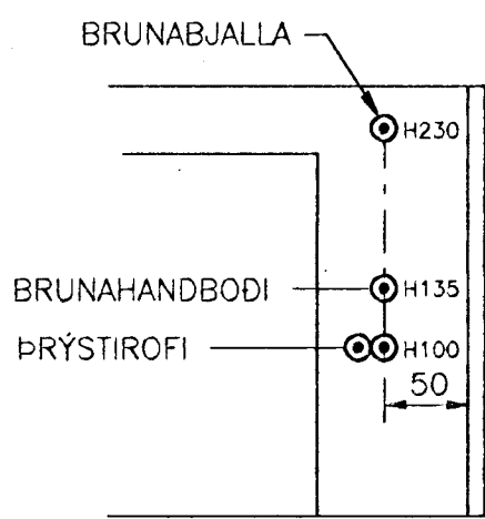
1:50 DÆMIGERD MYND FYRIR ALLAR HÆDIR
