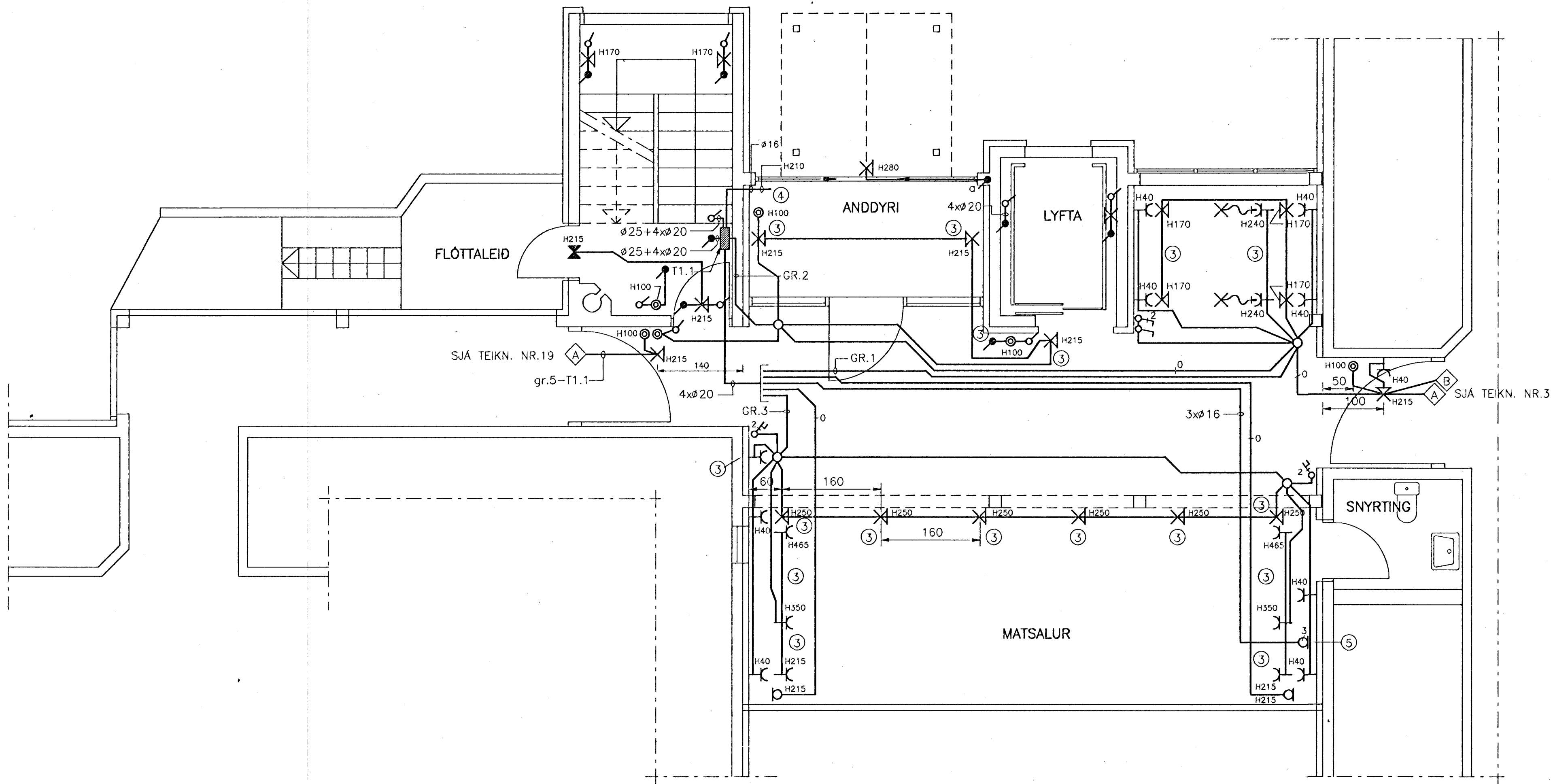
GRUNNMYND 1.HÆÐ TENGIBYGGING MKV: 1:50
