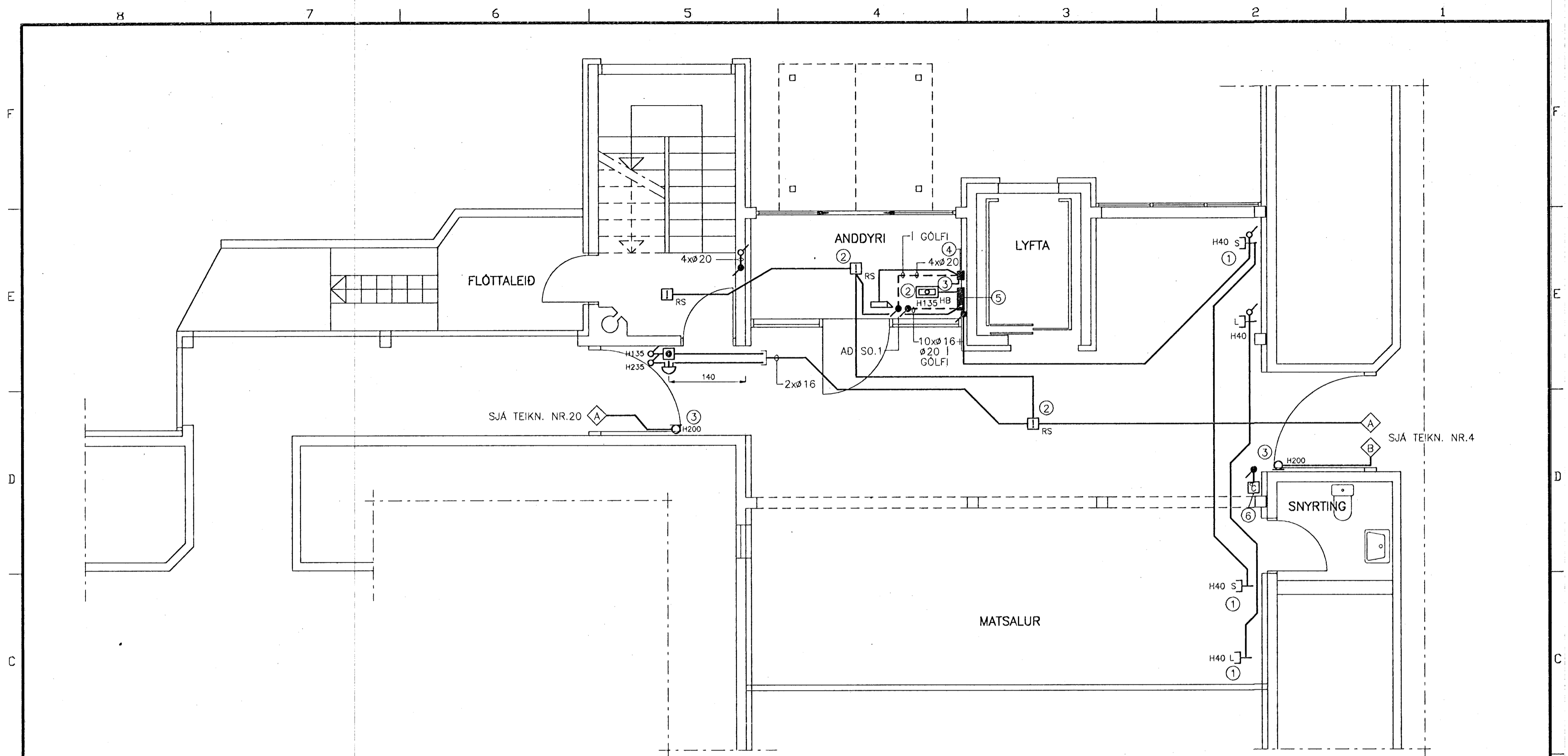
GRUNNMYND 1.HÆÐ TENGIÞYGGING MKV: 1:50
