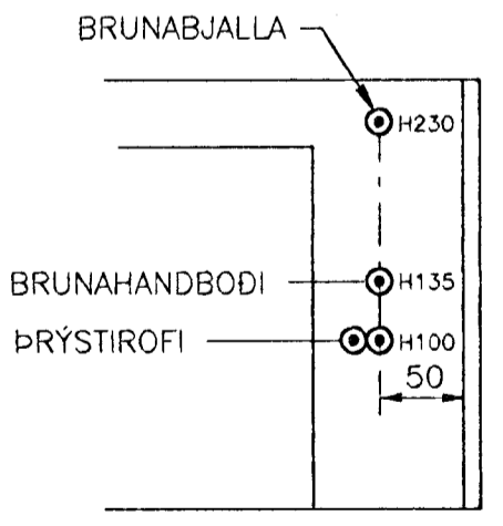
1:50 DÆMIGERD MYND FYRIR ALLAR HÆDIR
