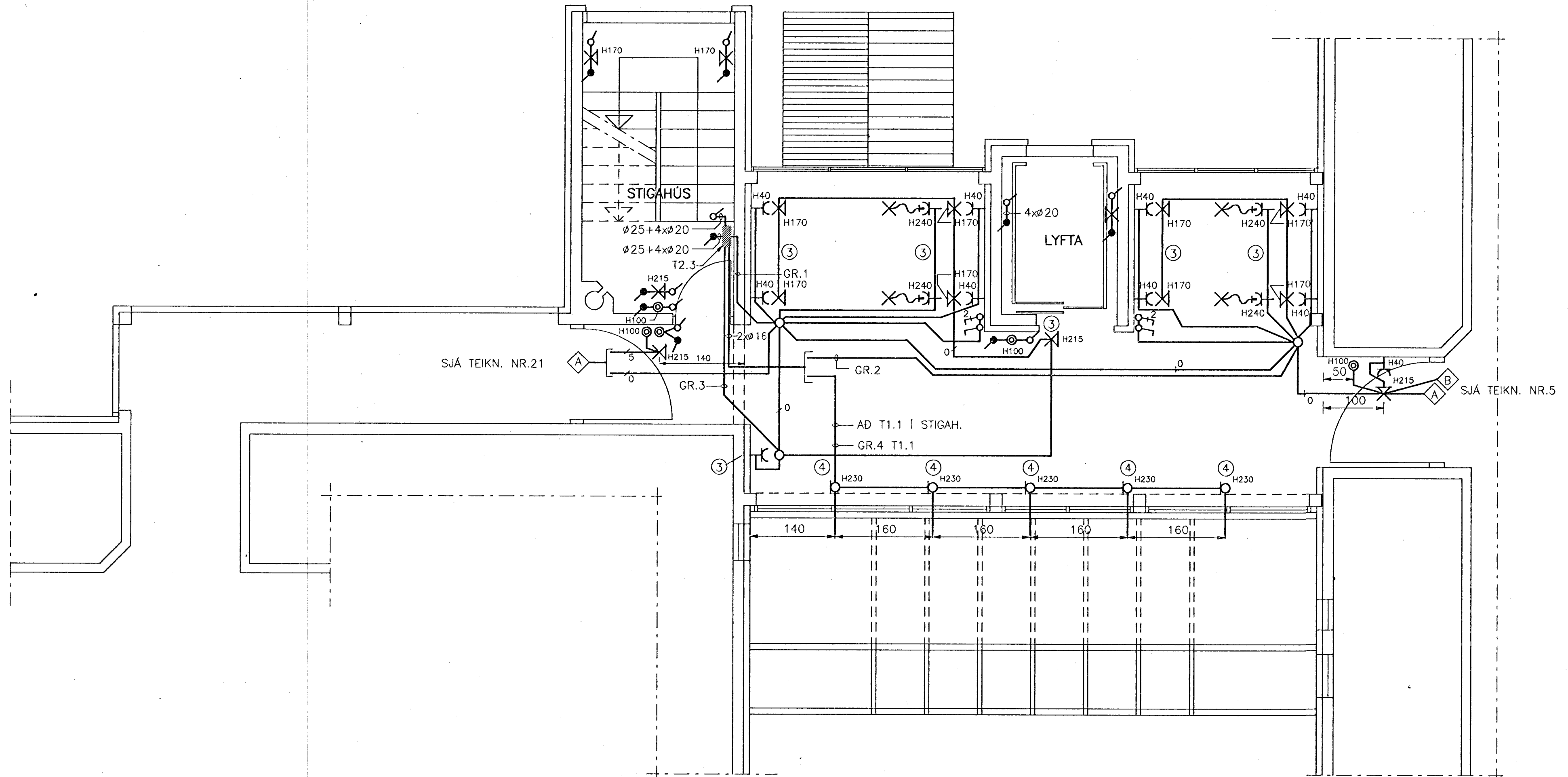
GRUNNMYND 2.HÆÐ TENGIBYGGING MKV: 1:50
