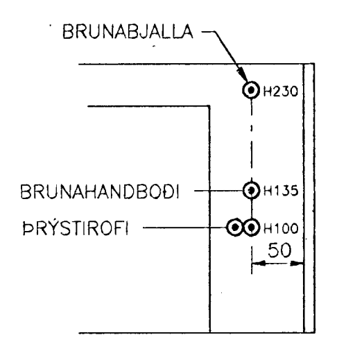
1:50 DÆMIGERD MYND FYRIR ALLAR HÆDIR
