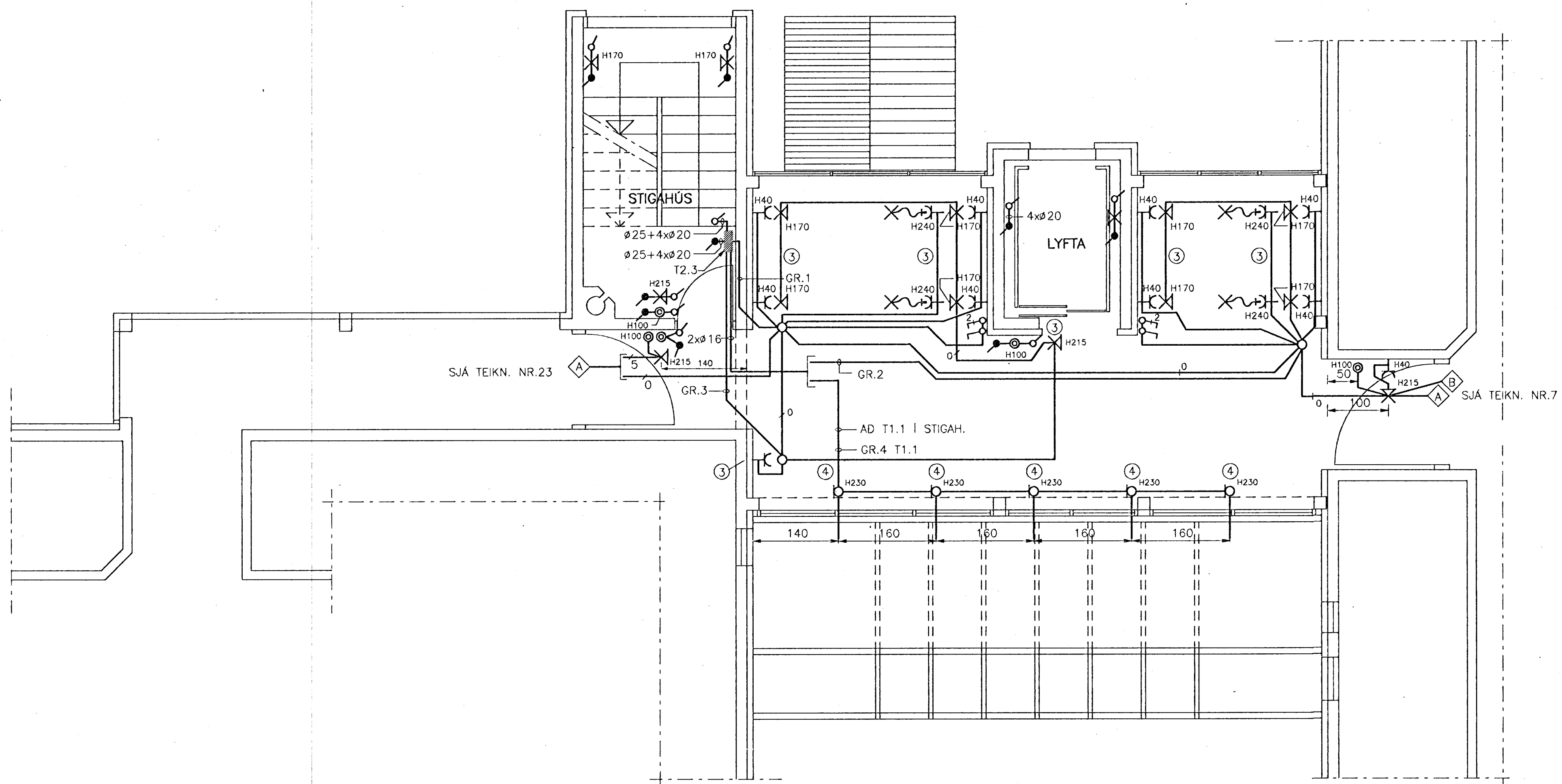
GRUNNMYND 3.HÆÐ TENGIÞYGGING MKV: 1:50
