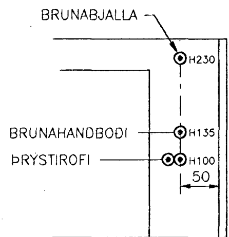
1:50 DÆMIGERÐ MYND FYRIR ALLAR HÆÐIR
