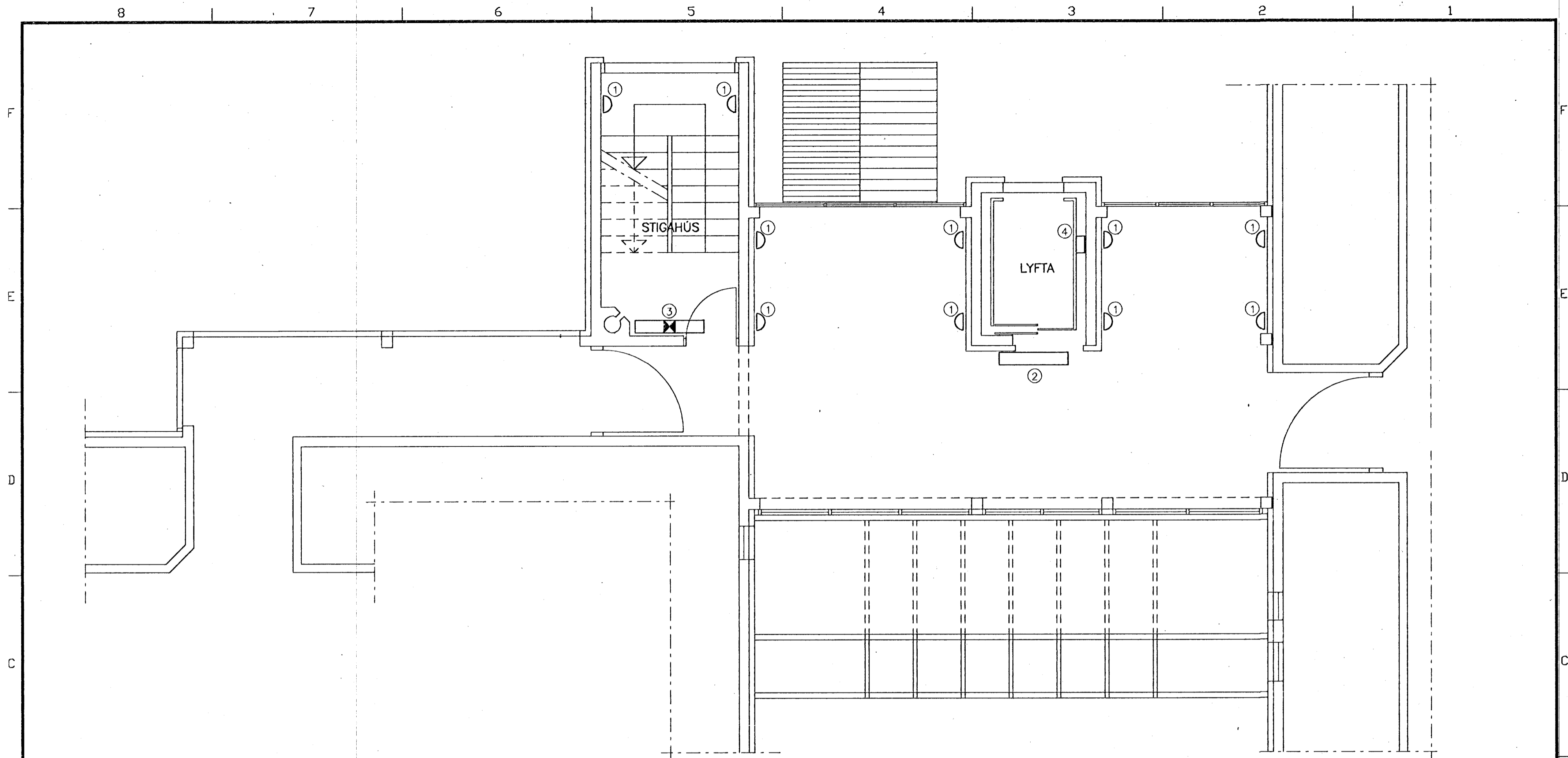
GRUNNMYND 3.HÆÐ TENGIÐBYGGING MKV: 1:50
