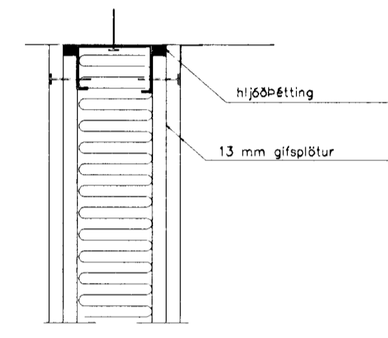
LÓDRÉTT DEILI GIFS VEGGUR - FRÁGANGUR VÍÐ BITA Í LOFTI
