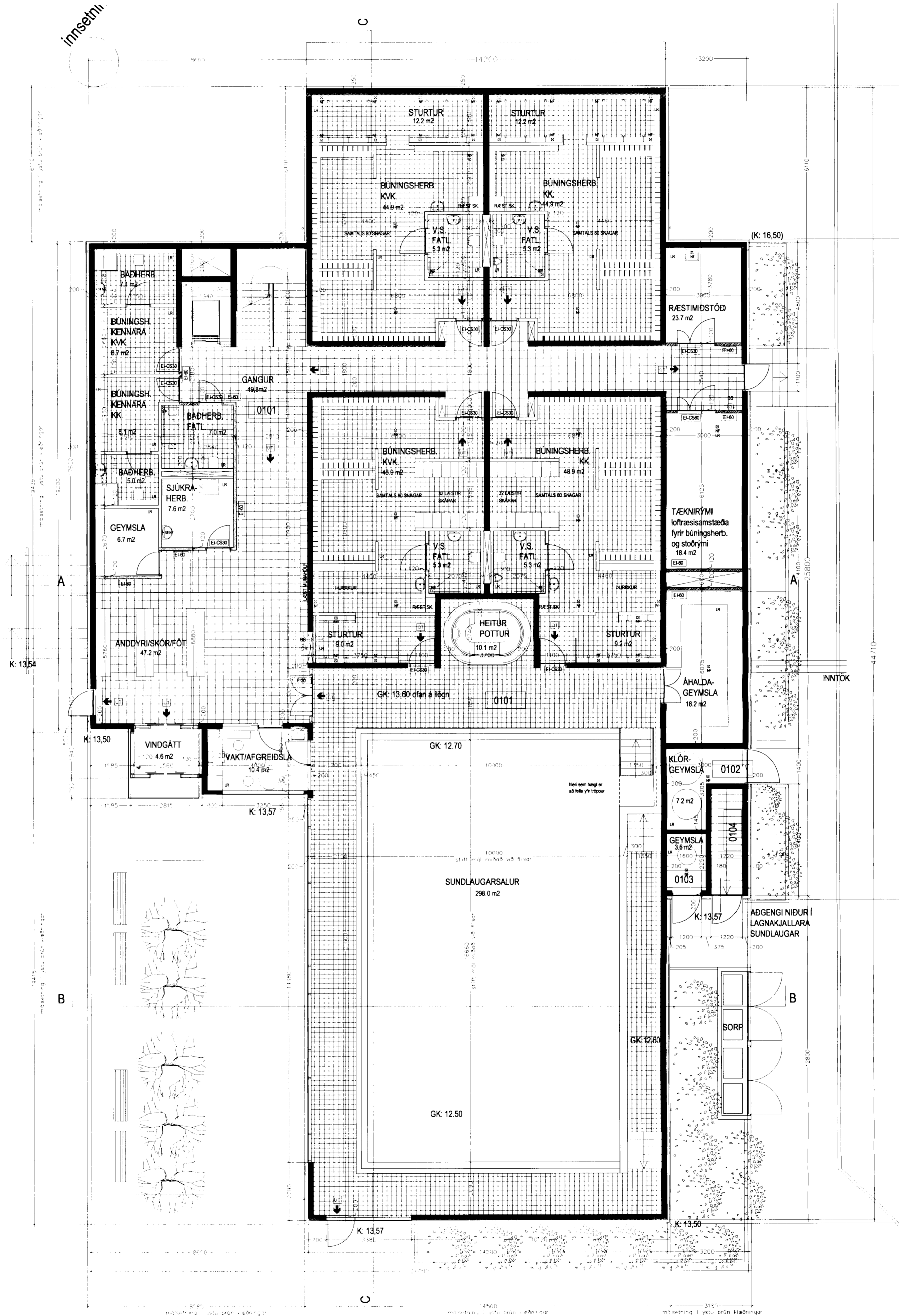
GRUNNMYND 1. HÆÐAR
